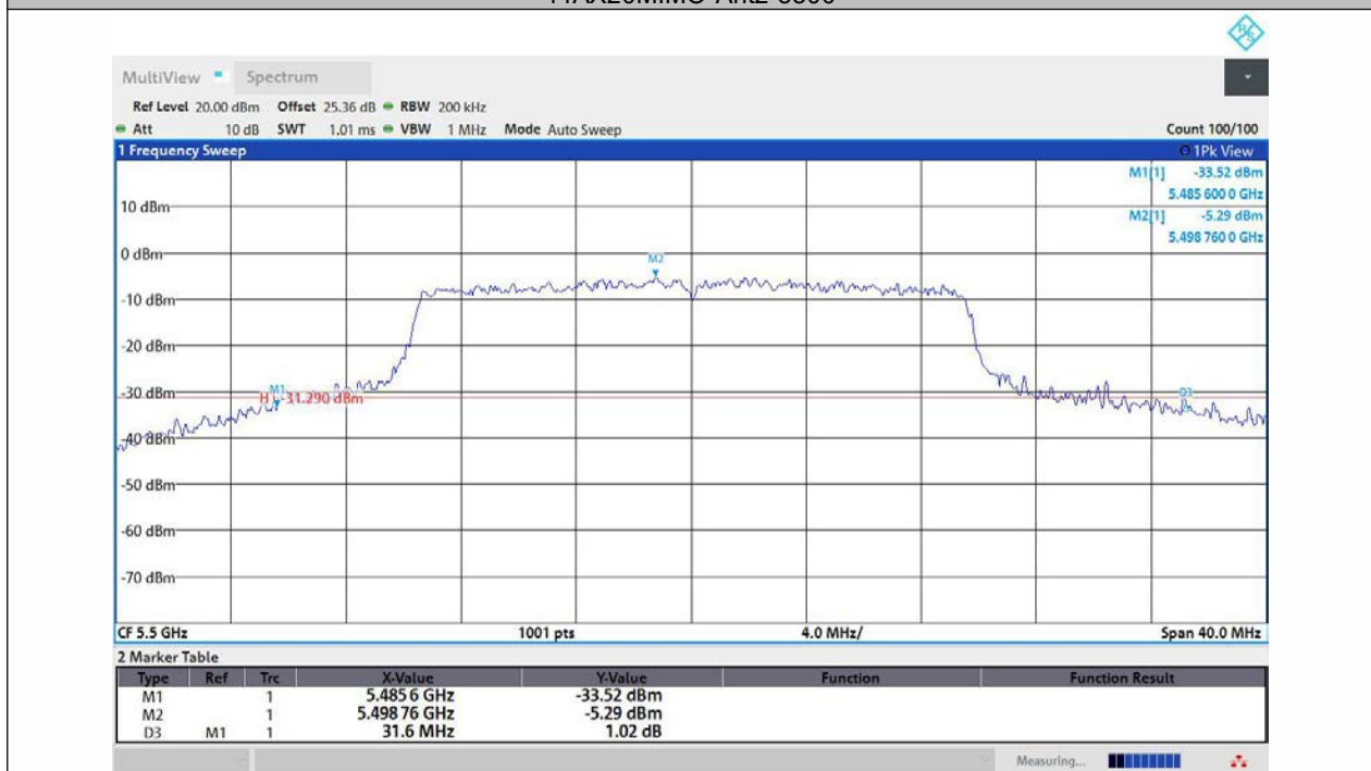
11AX20MIMO-Ant3-5500
