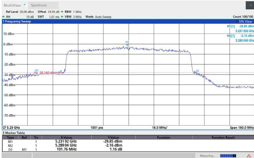
11AX80MIMO-Ant3-5290
