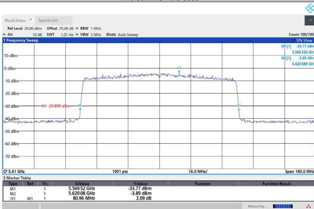
11AX80MIMO-Ant1-5610
