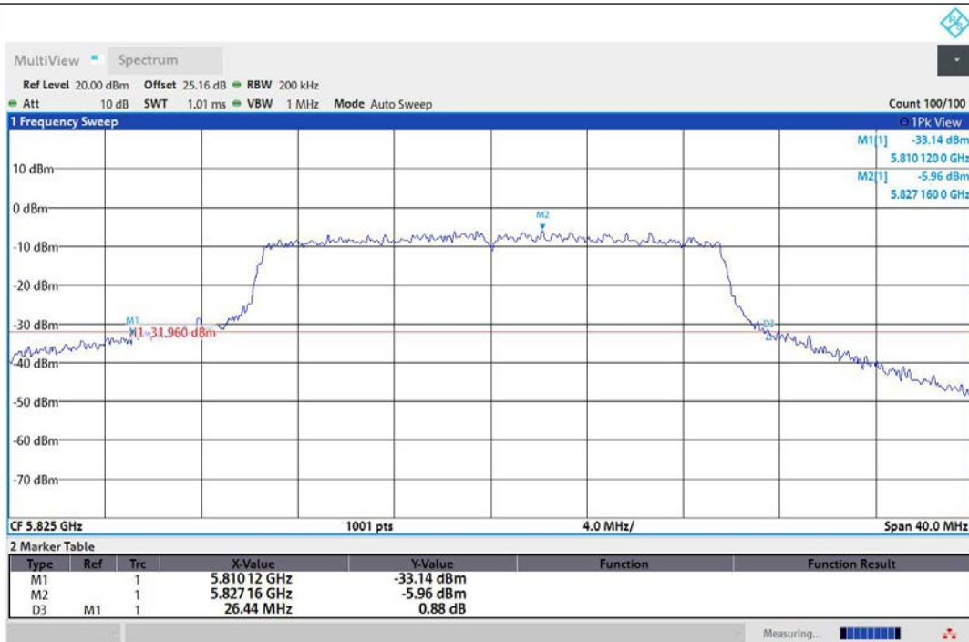
11AX20MIMO-Ant1-5825
