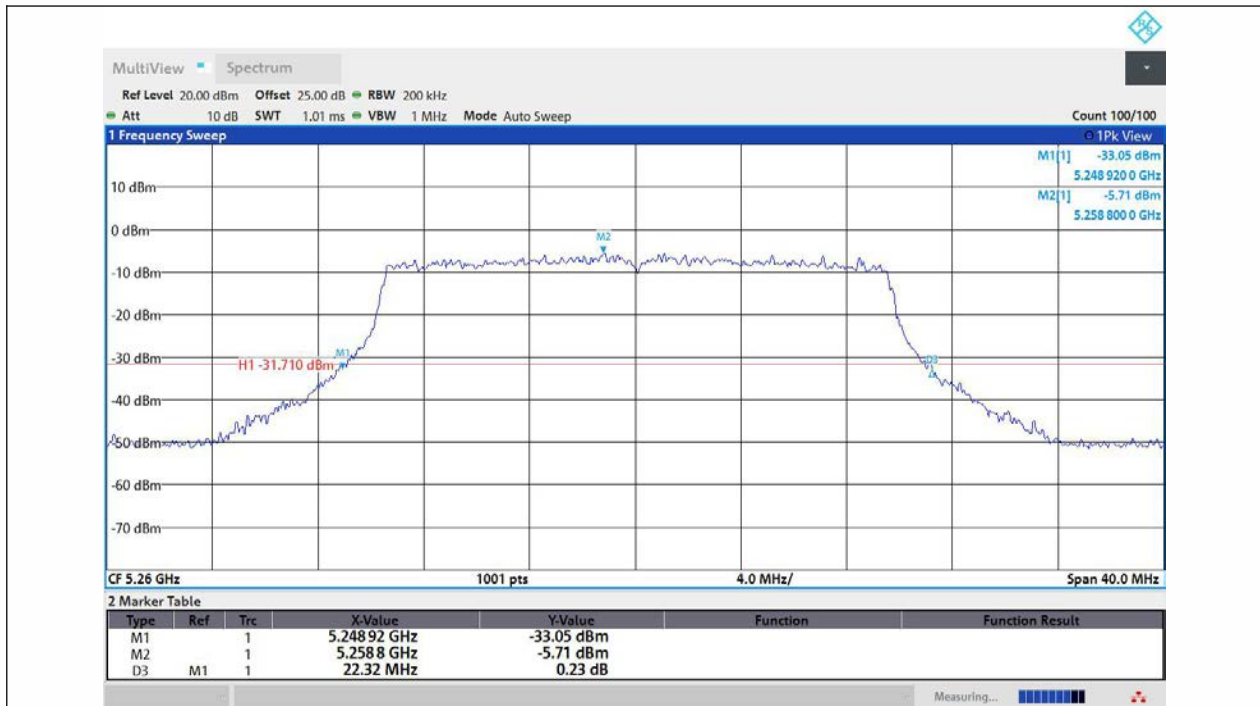
11AX20MIMO-Ant1-5260
