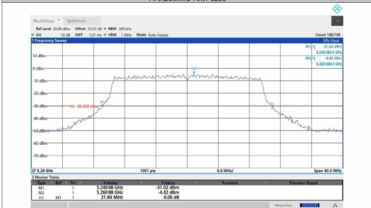
11AX20MIMO-Ant2-5260
