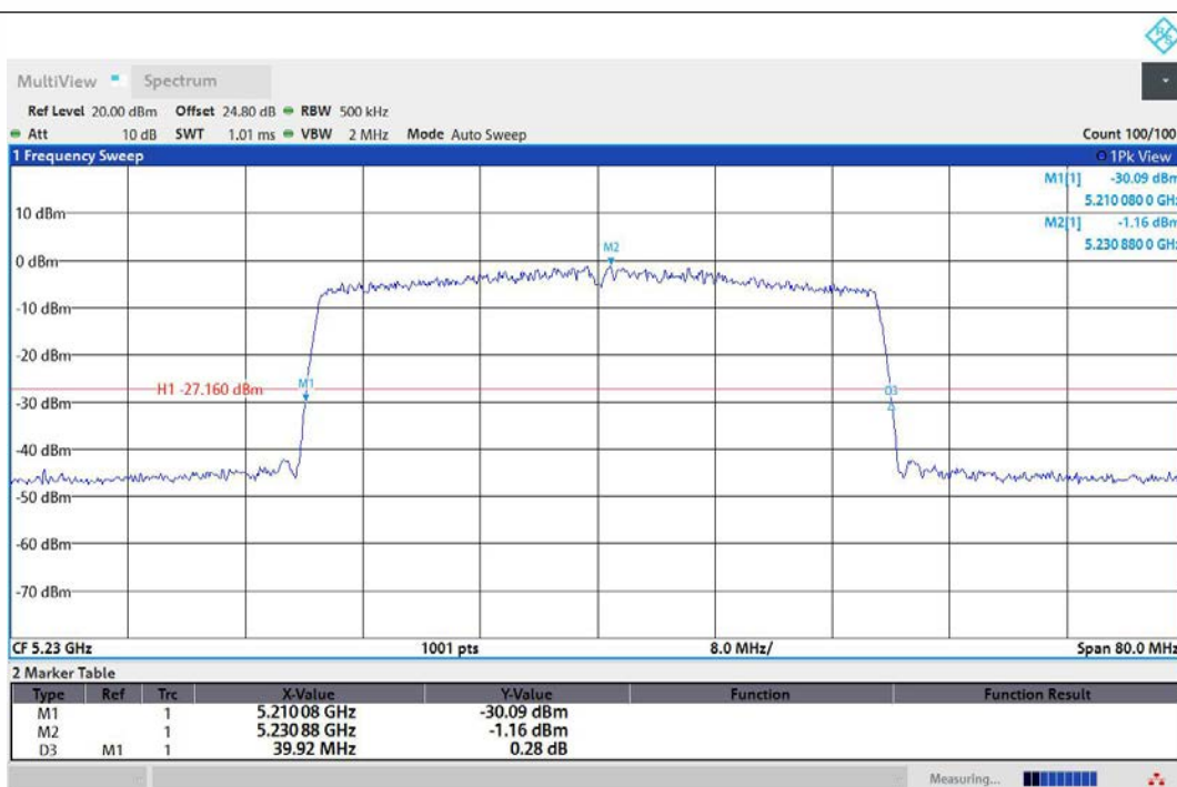
11AX40MIMO-Ant3-5230
