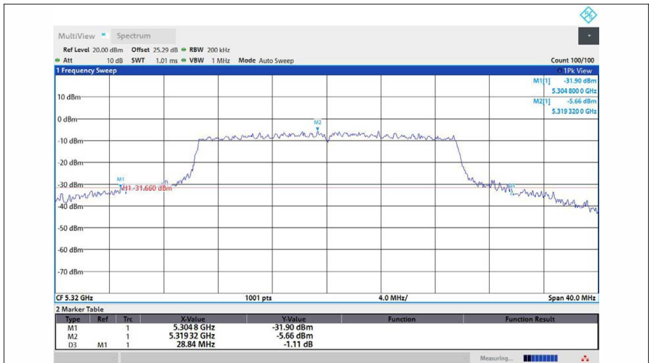
11AX20MIMO-Ant3-5320
