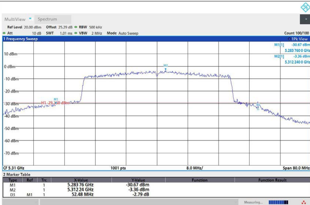
11AX40MIMO-Ant1-5310
