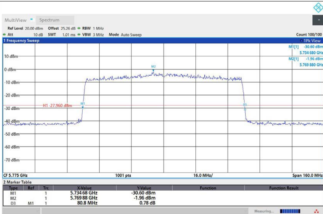
11AX80MIMO-Ant1-5775
