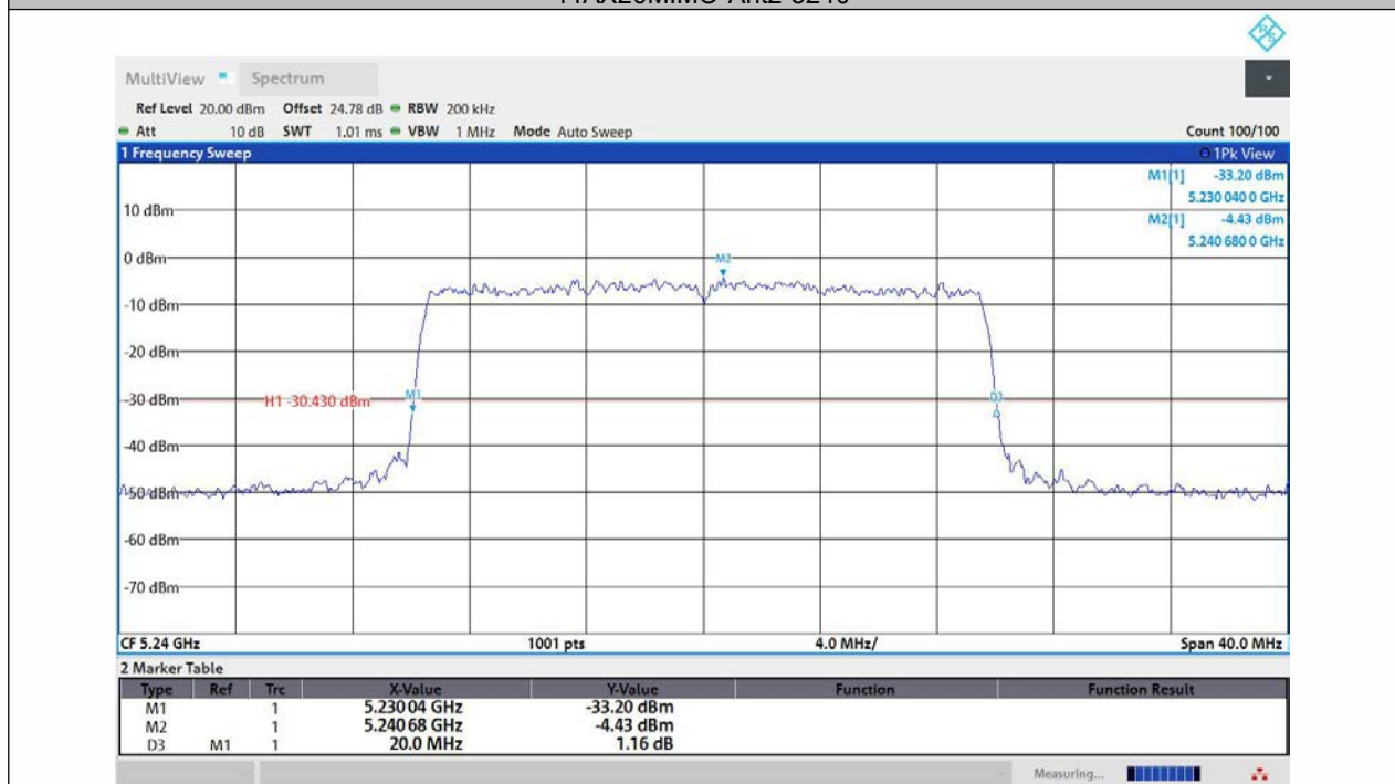
11AX20MIMO-Ant3-5240
