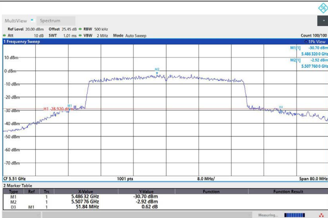
11AX40MIMO-Ant1-5510
