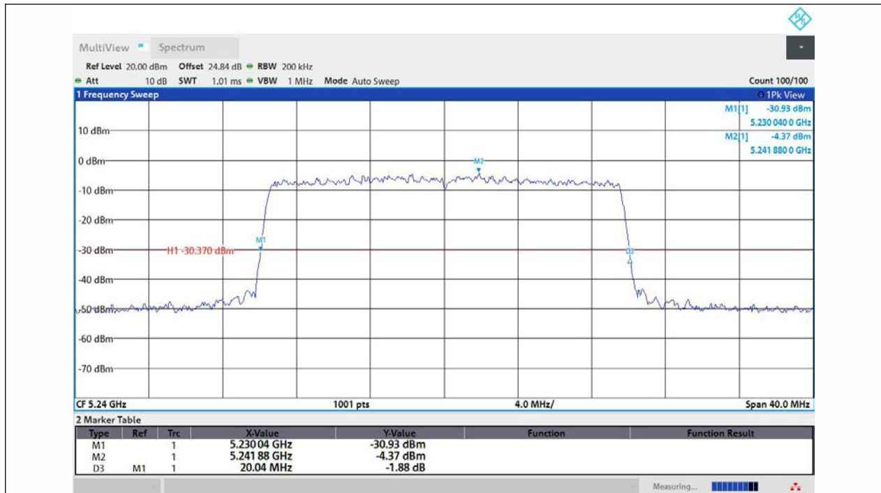
11AX20MIMO-Ant2-5240
