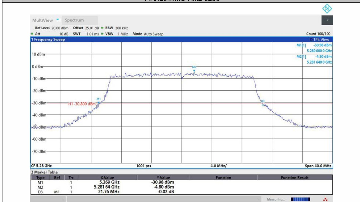
11AX20MIMO-Ant3-5280
