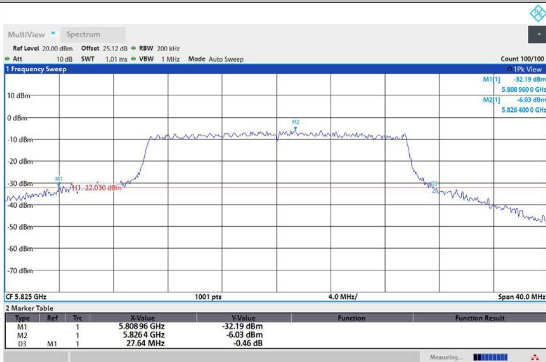
11AX20MIMO-Ant2-5825
