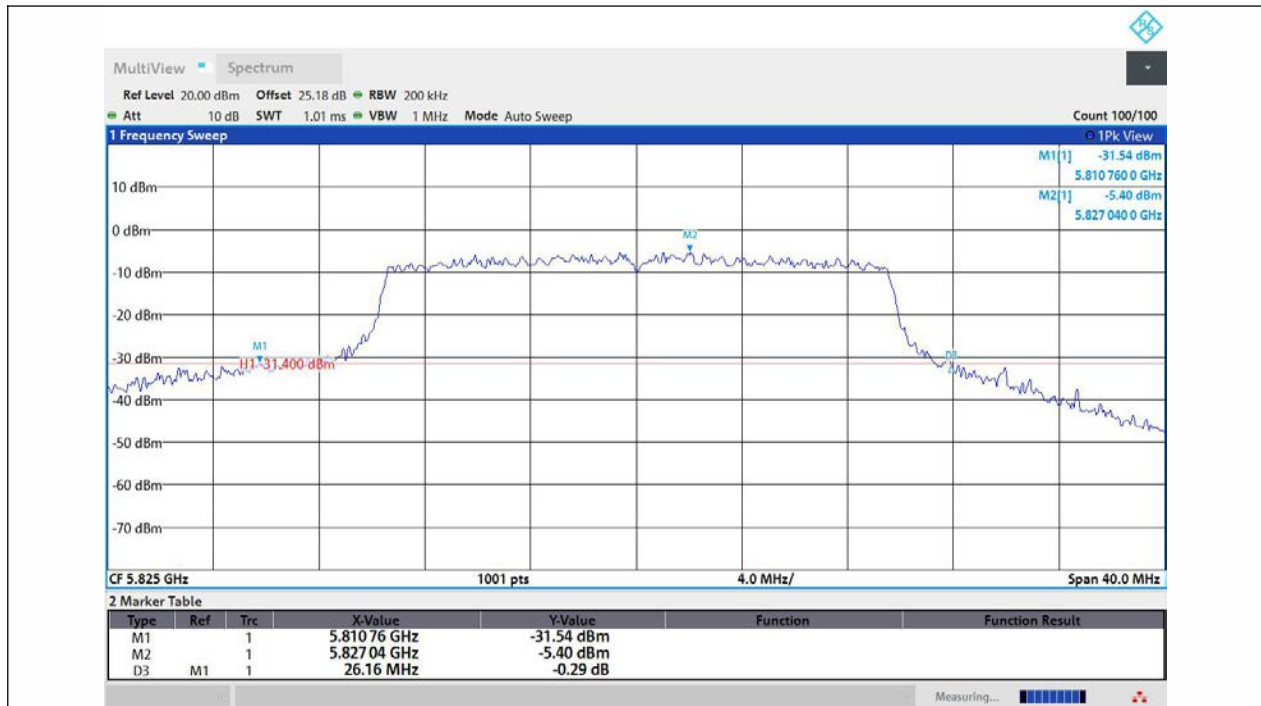
11AX20MIMO-Ant3-5825
