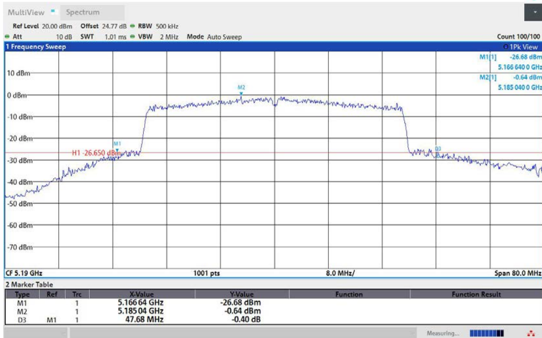
11AX40MIMO-Ant3-5190
