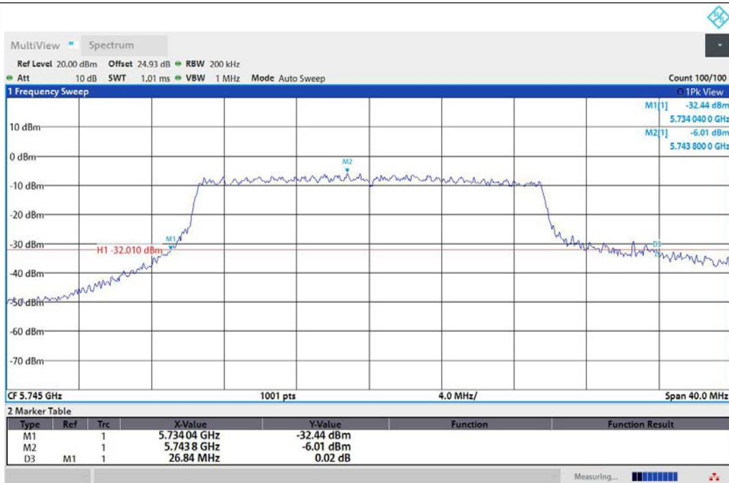
11AX20MIMO-Ant3-5745
