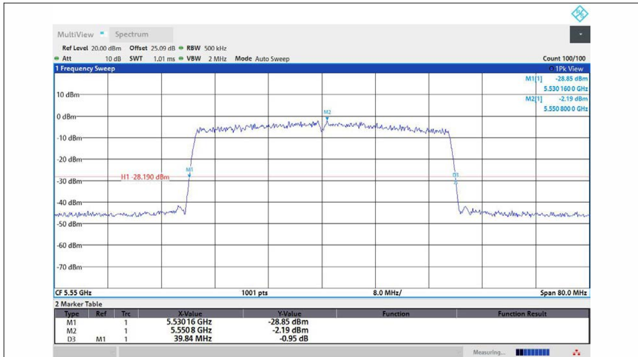
11AX40MIMO-Ant3-5550
