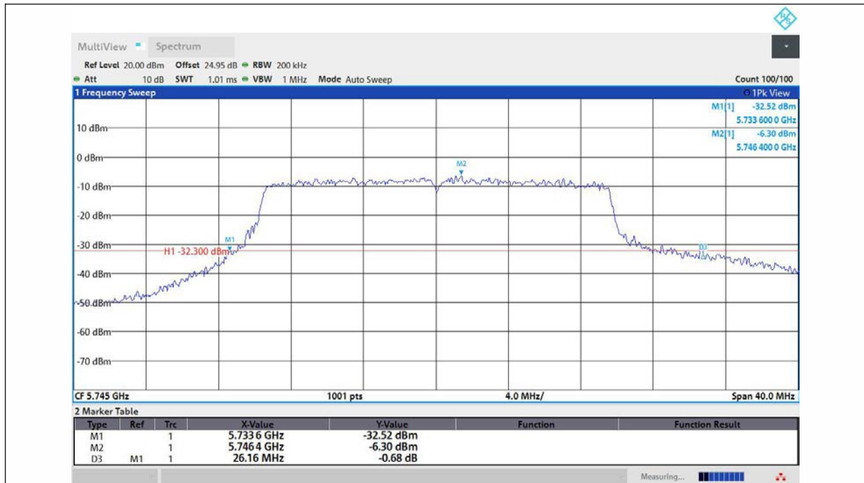
11AX20MIMO-Ant1-5745
