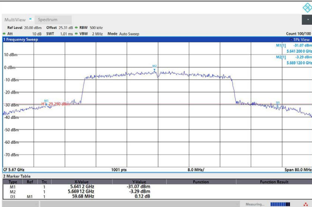
11AX40MIMO-Ant3-5670
