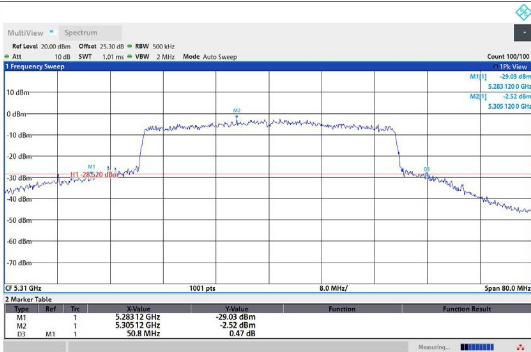
11AX40MIMO-Ant3-5310
