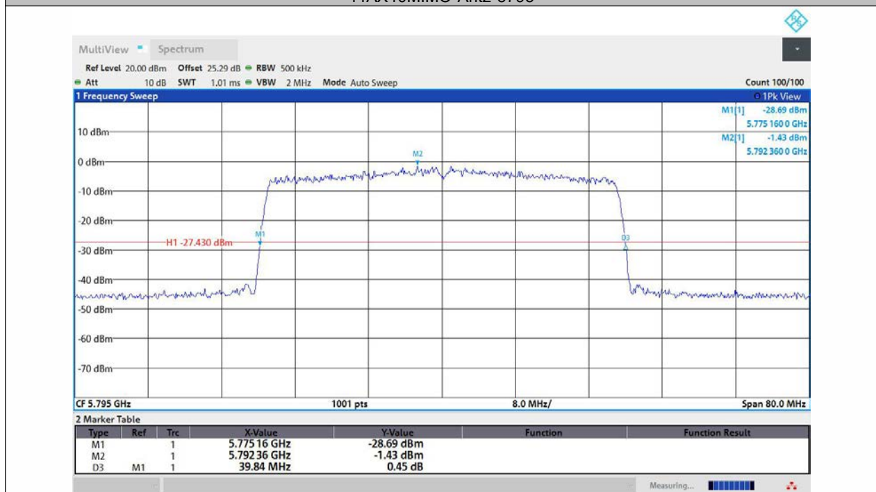
11AX40MIMO-Ant3-5795
