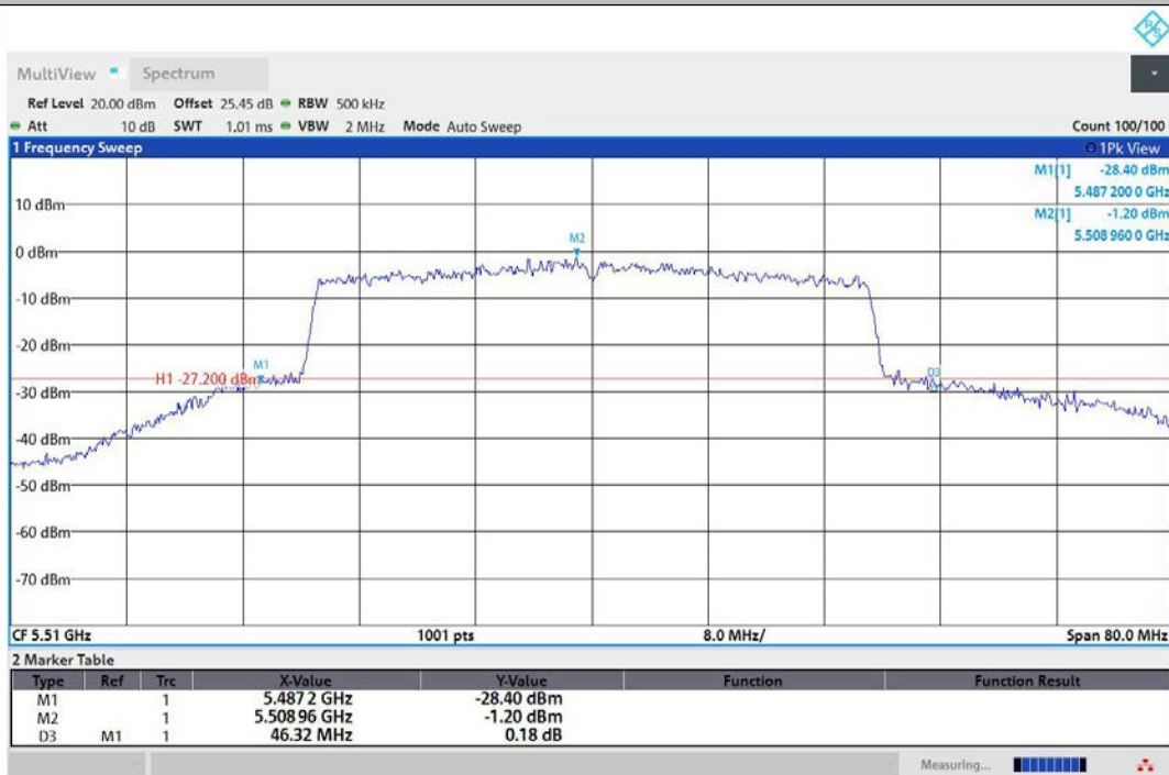
11AX40MIMO-Ant3-5510
