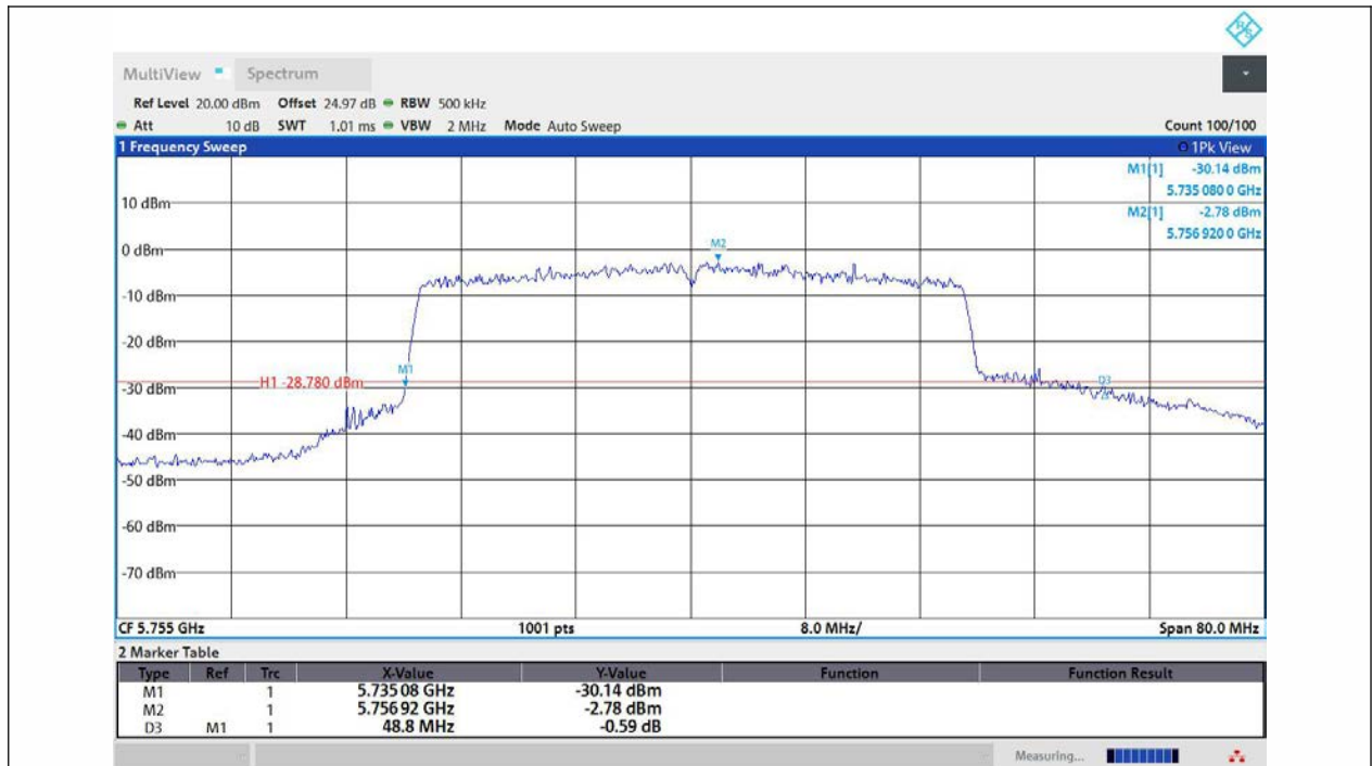
11AX40MIMO-Ant3-5755
