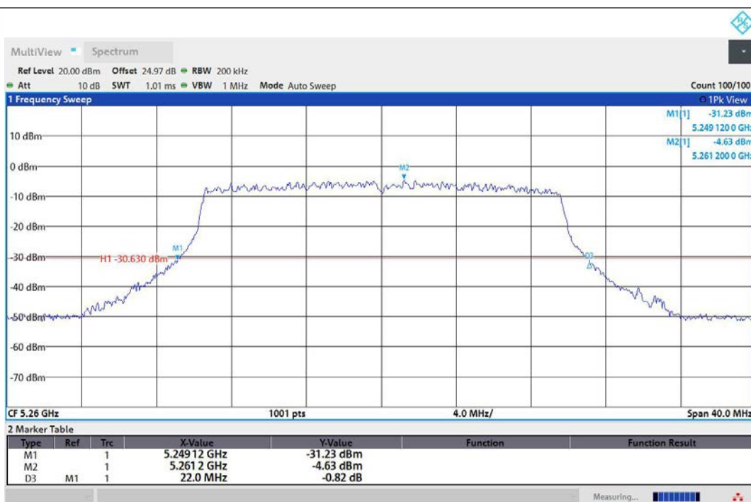
11AX20MIMO-Ant3-5260
