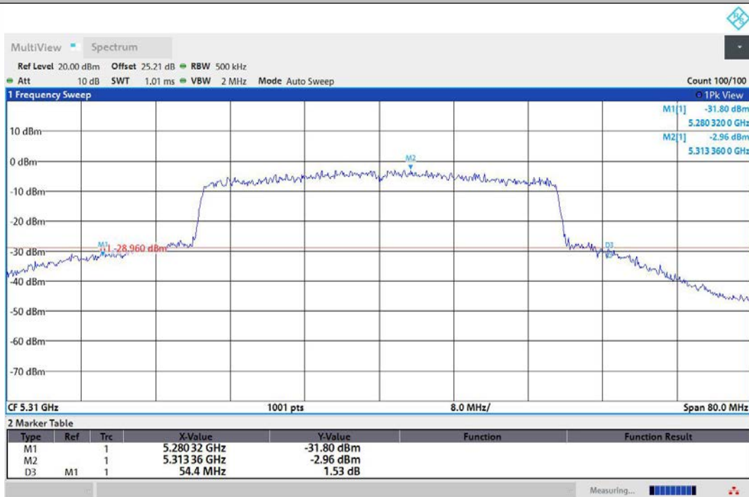
11AX40MIMO-Ant2-5310
