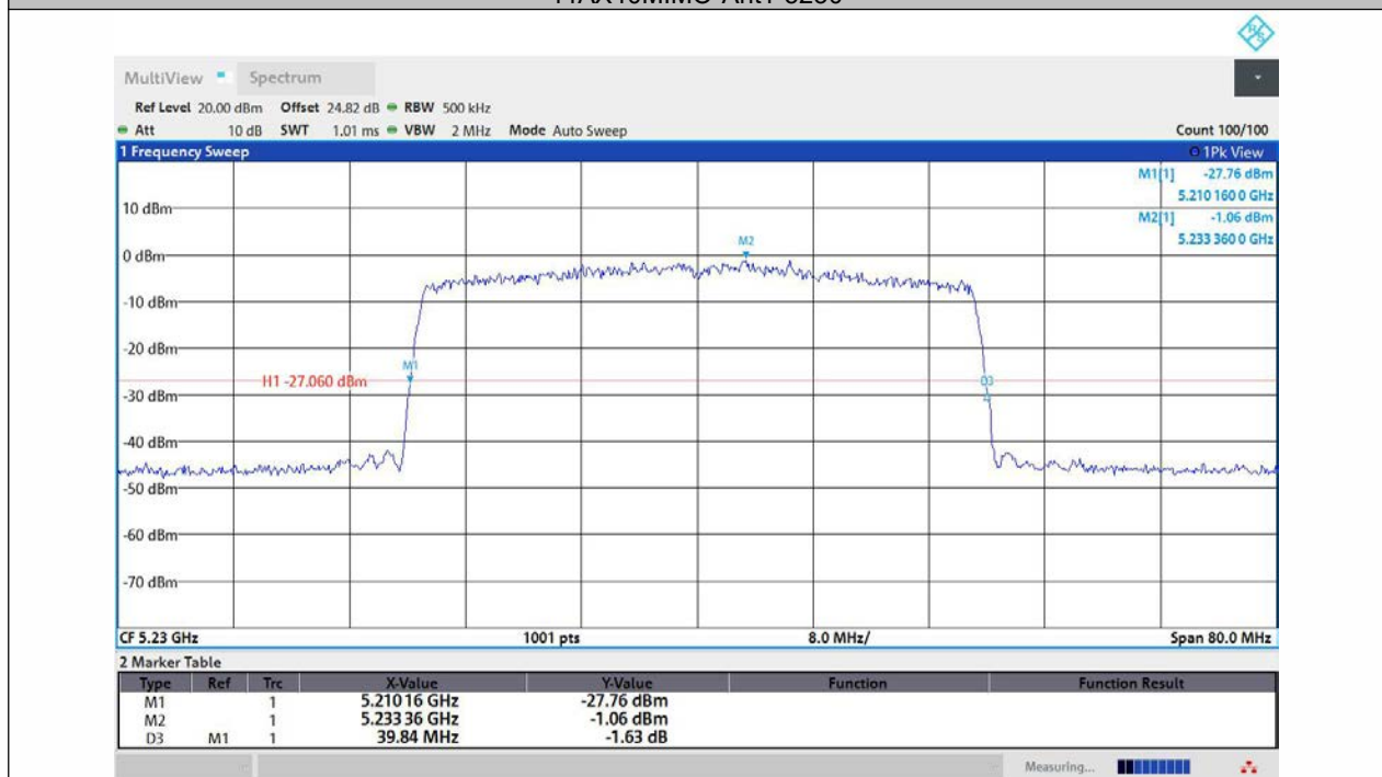
11AX40MIMO-Ant2-5230
