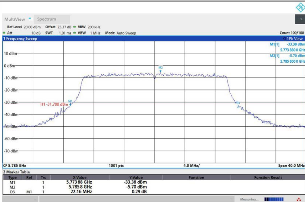
11AX20MIMO-Ant1-5785
