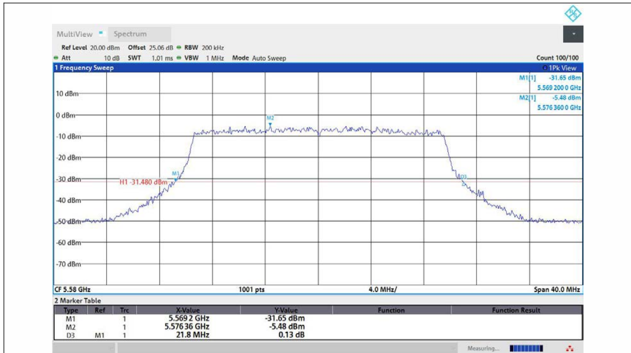
11AX20MIMO-Ant3-5580
