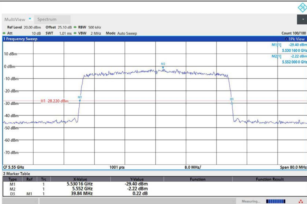
11AX40MIMO-Ant2-5550
