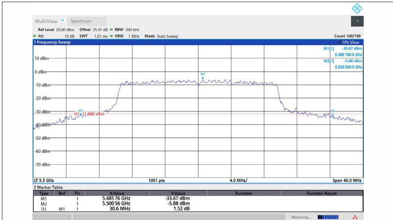
11AX20MIMO-Ant2-5500
