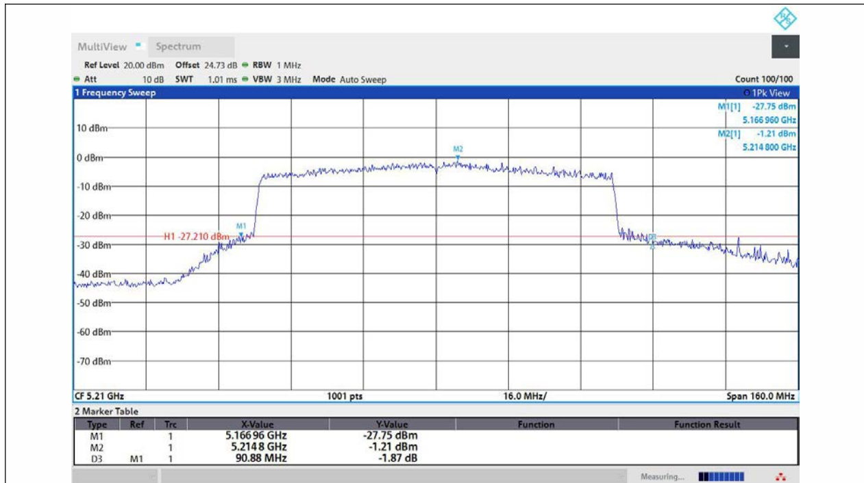
11AX80MIMO-Ant3-5210
