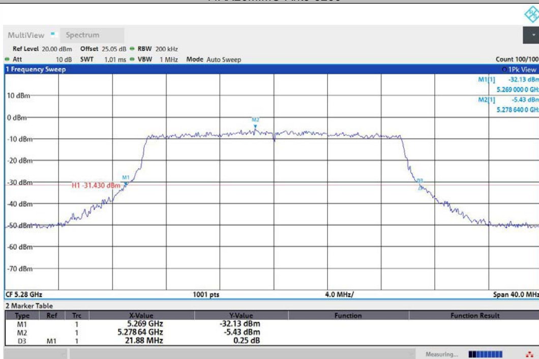
11AX20MIMO-Ant1-5280
