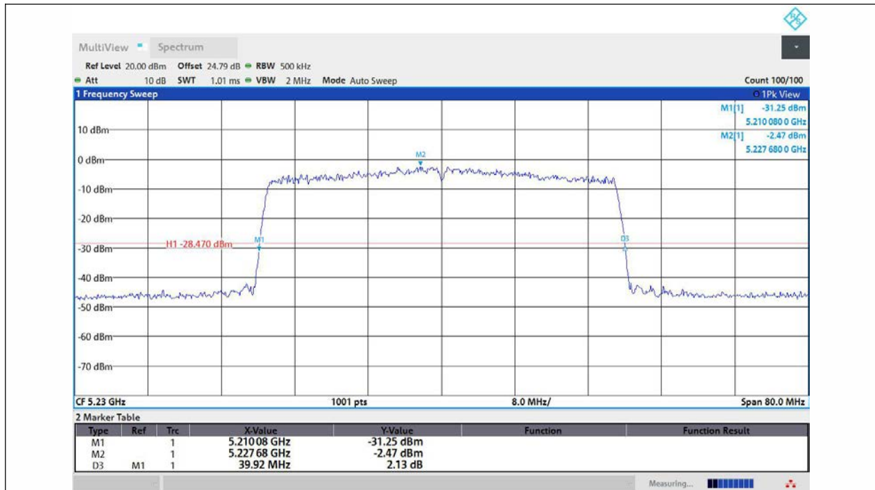
11AX40MIMO-Ant1-5230
