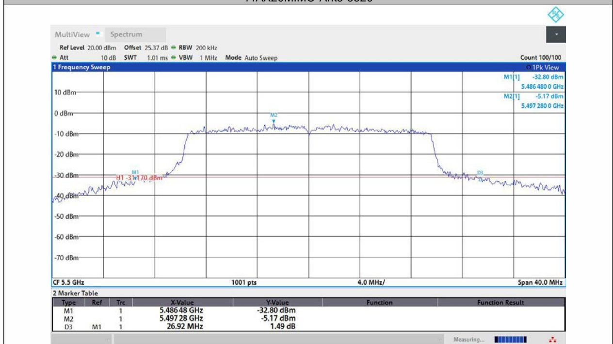
11AX20MIMO-Ant1-5500
