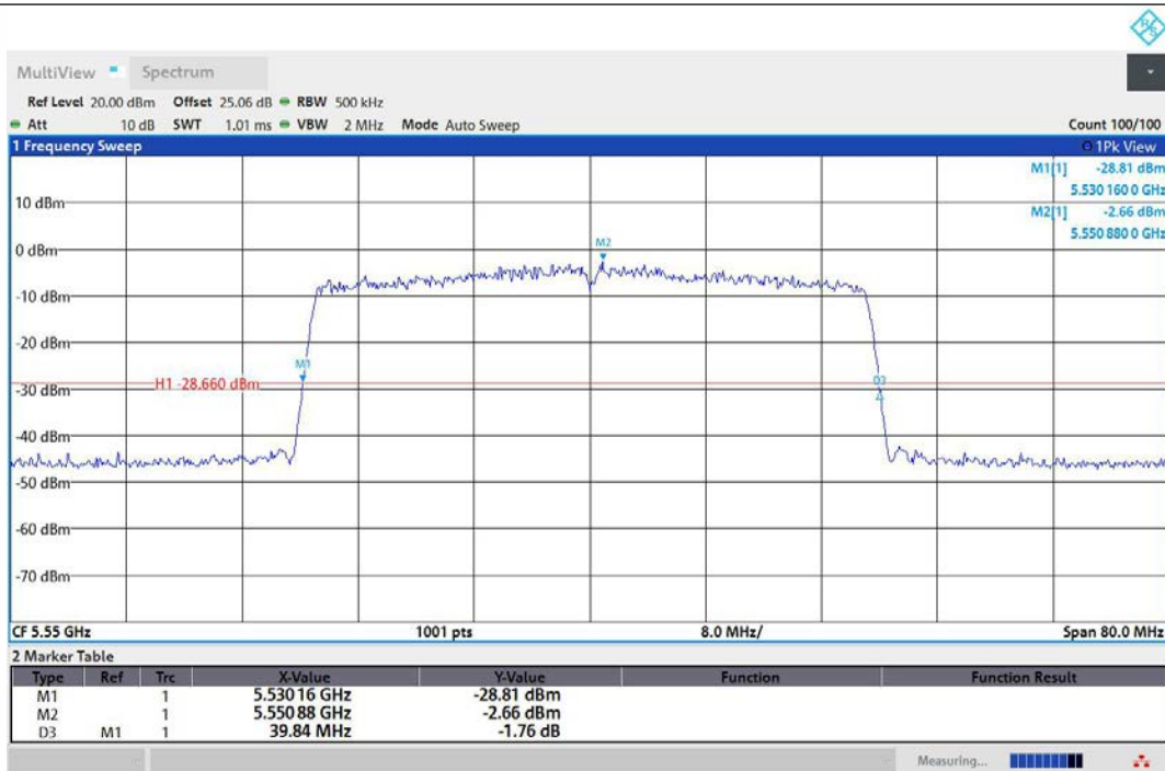
11AX40MIMO-Ant1-5550
