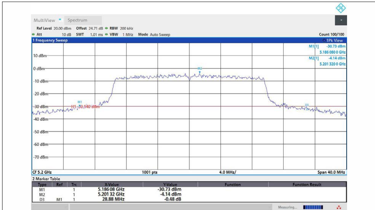
11AX20MIMO-Ant3-5200
