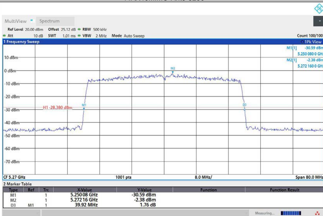
11AX40MIMO-Ant1-5270
