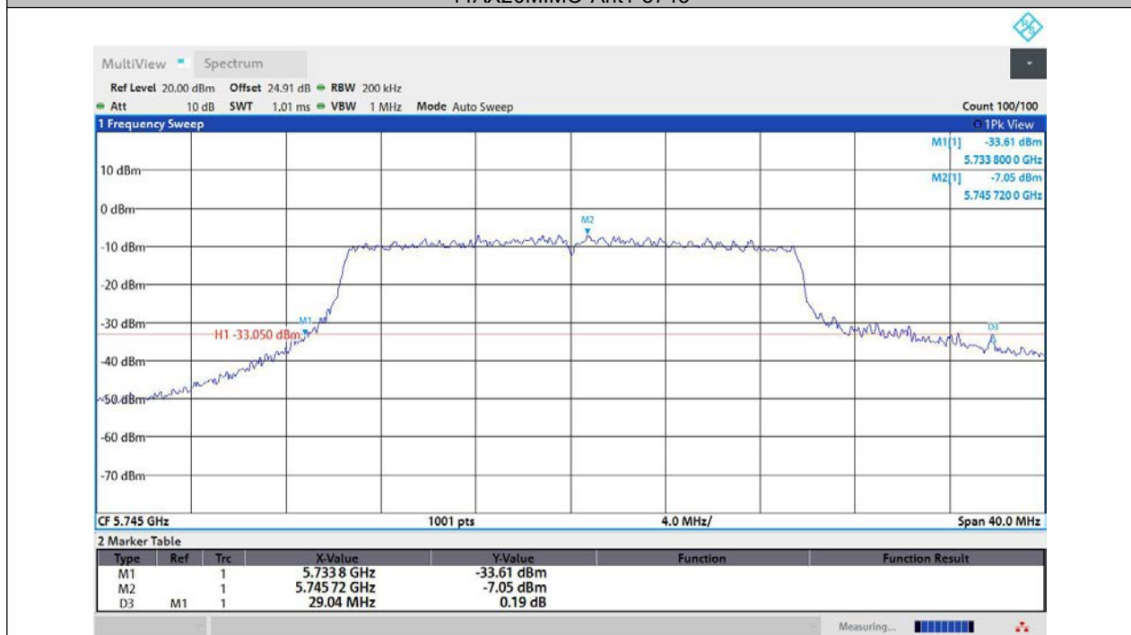
11AX20MIMO-Ant2-5745
