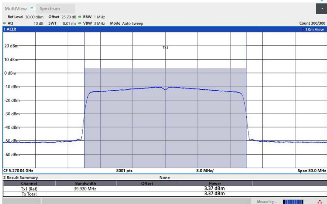
11AX40MIMO-Ant1-5270-TPC_H-PASS
