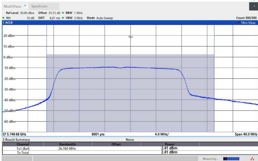
11AX20MIMO-Ant1-5745-PASS
