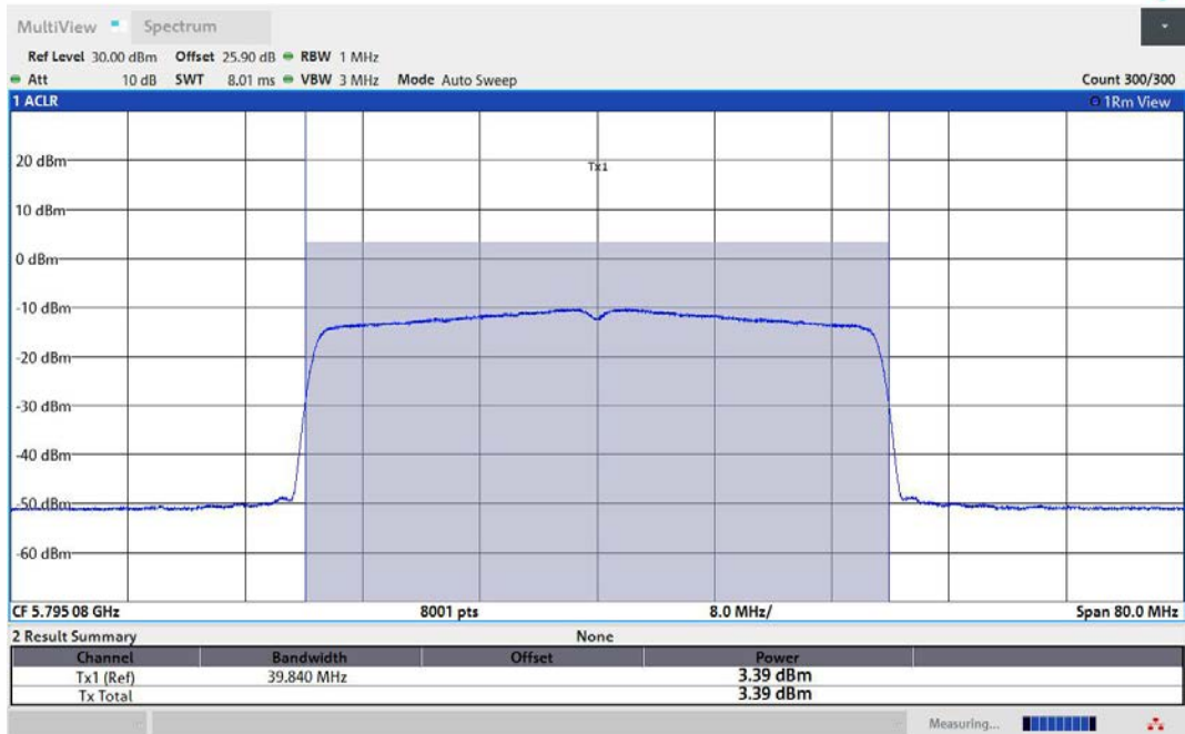
11AX40MIMO-Ant1-5795-PASS
