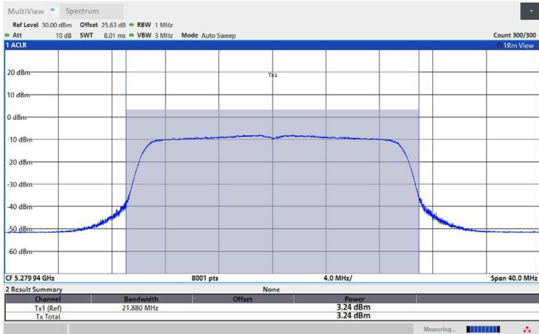
11AX20MIMO-Ant1-5280-TPC_H-PASS
