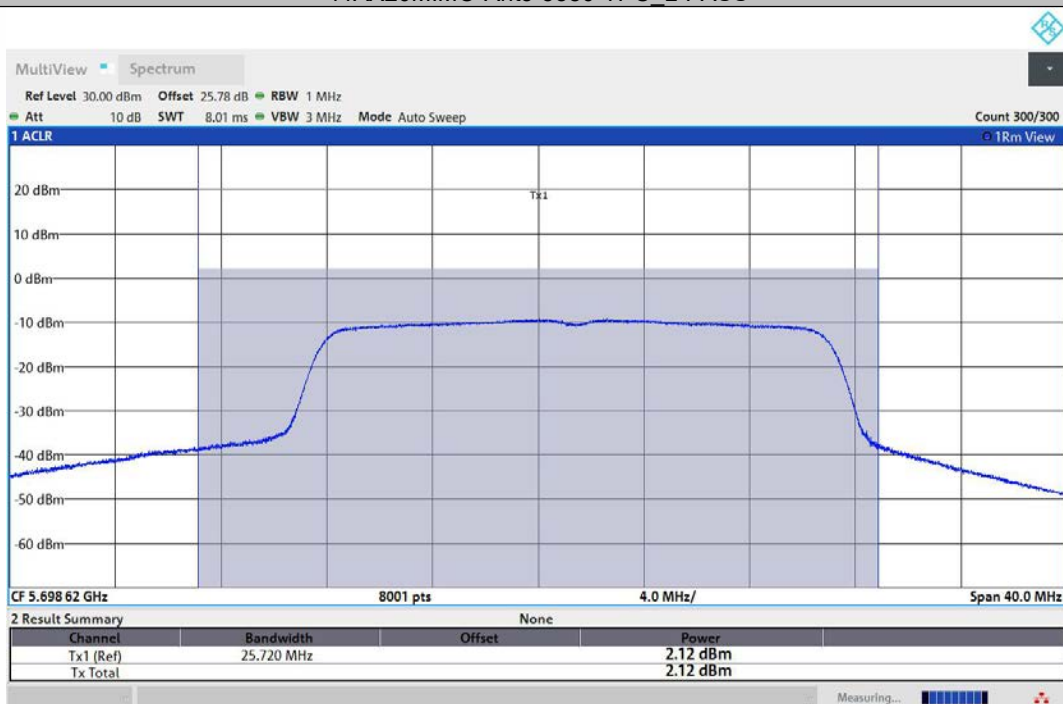
11AX20MIMO-Ant1-5700-TPC_H-PASS
