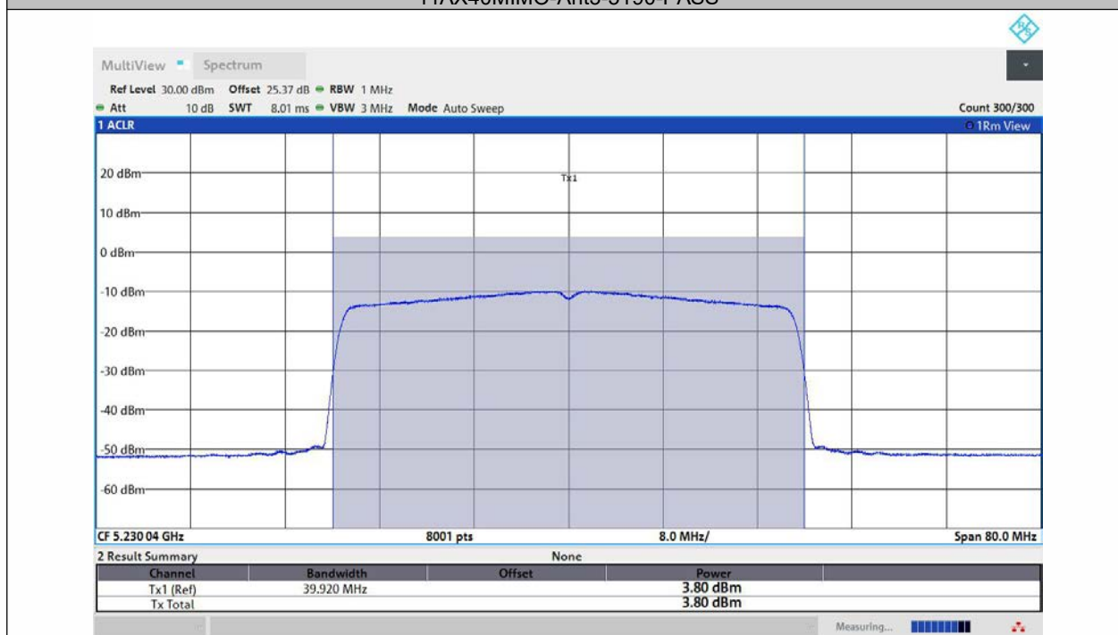
11AX40MIMO-Ant1-5230-PASS
