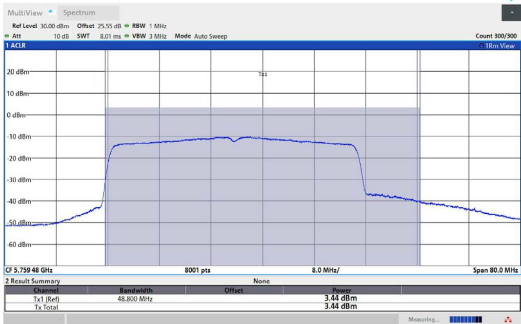
11AX40MIMO-Ant3-5755-PASS
