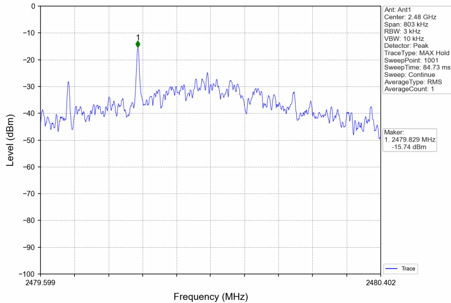
1M_HCH_2480MHz_DataRate=_Ant1_NTNV
