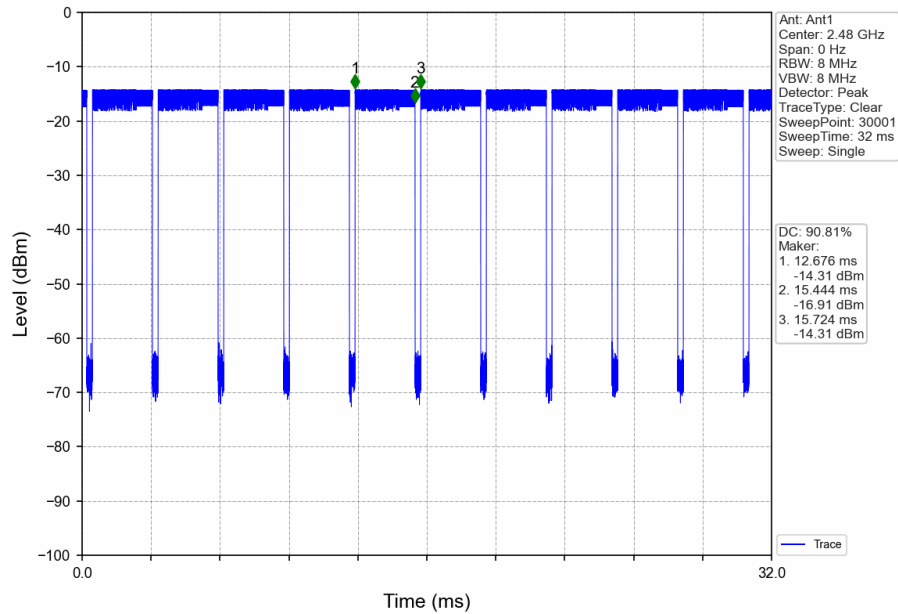
1M_HCH_2480MHz_DataRate=_Ant1_NTNV
