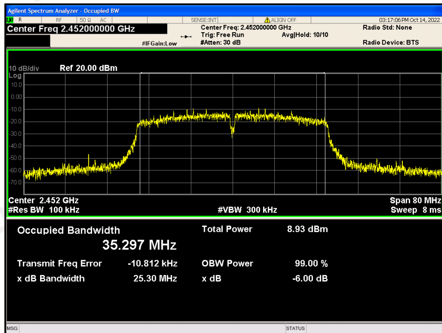
CH09: 2452MHz
