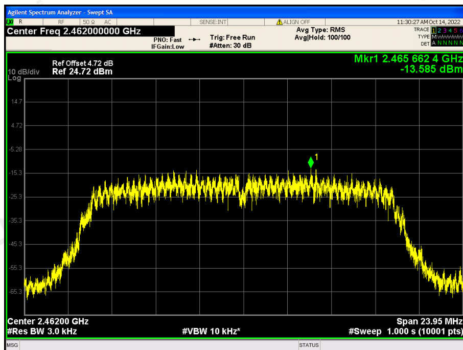
CH11: 2462MHz
