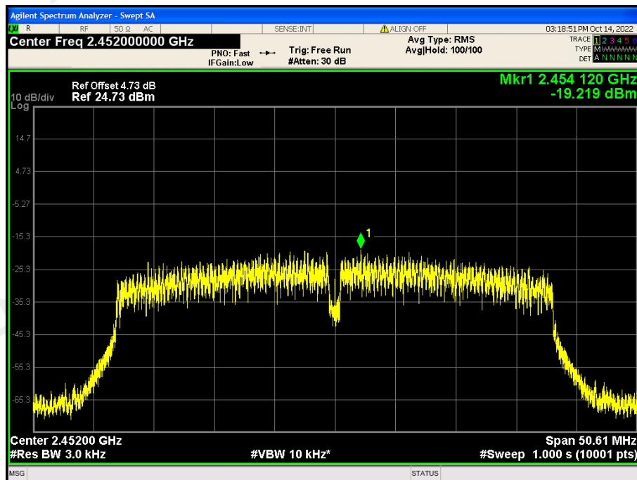
CH09: 2452MHz
