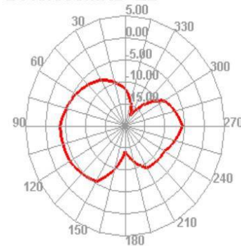
2440.000MHz E2
