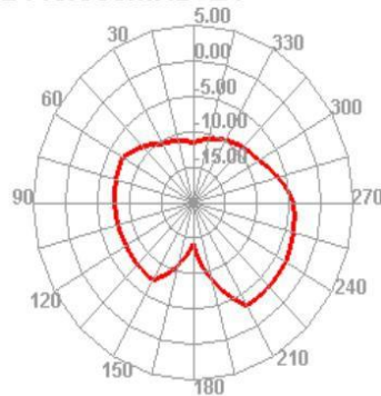
2440.000MHz E1
