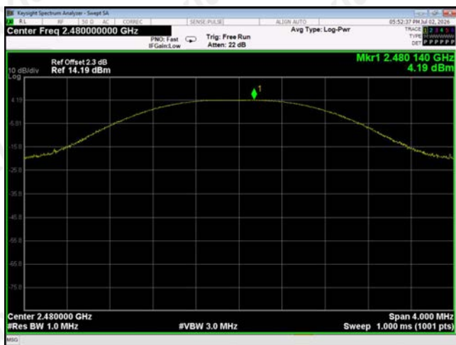
GFSK(CH78)
