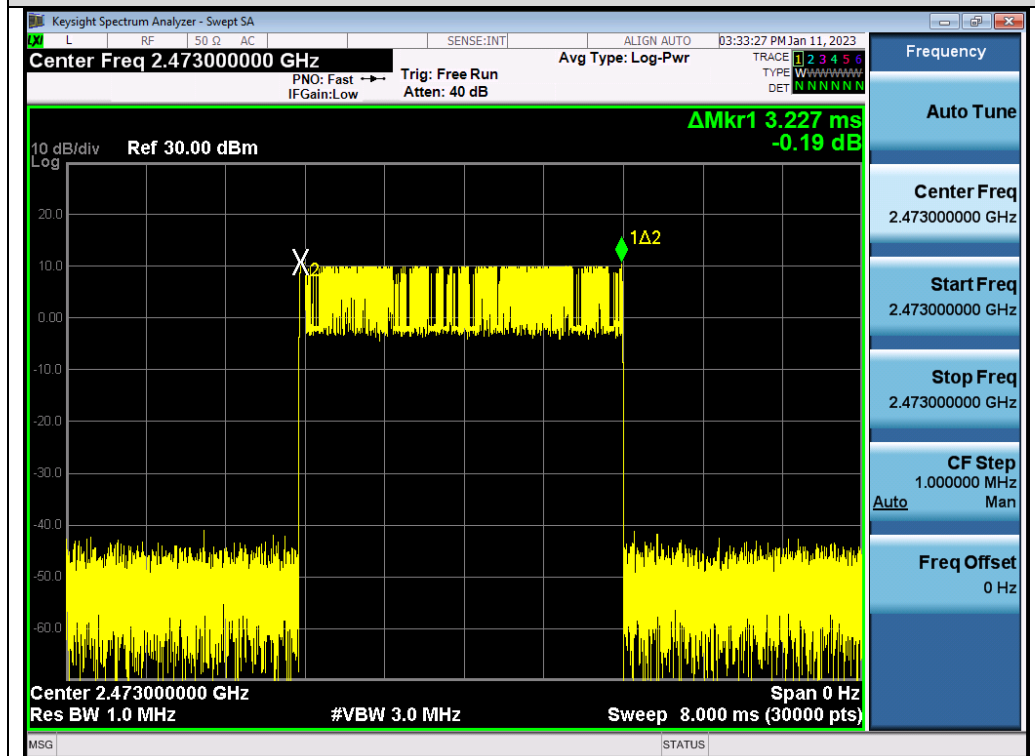
Test_Graph_2.4G_HOP_ANT1_NA_4Mbps_2473_Time per Burst
