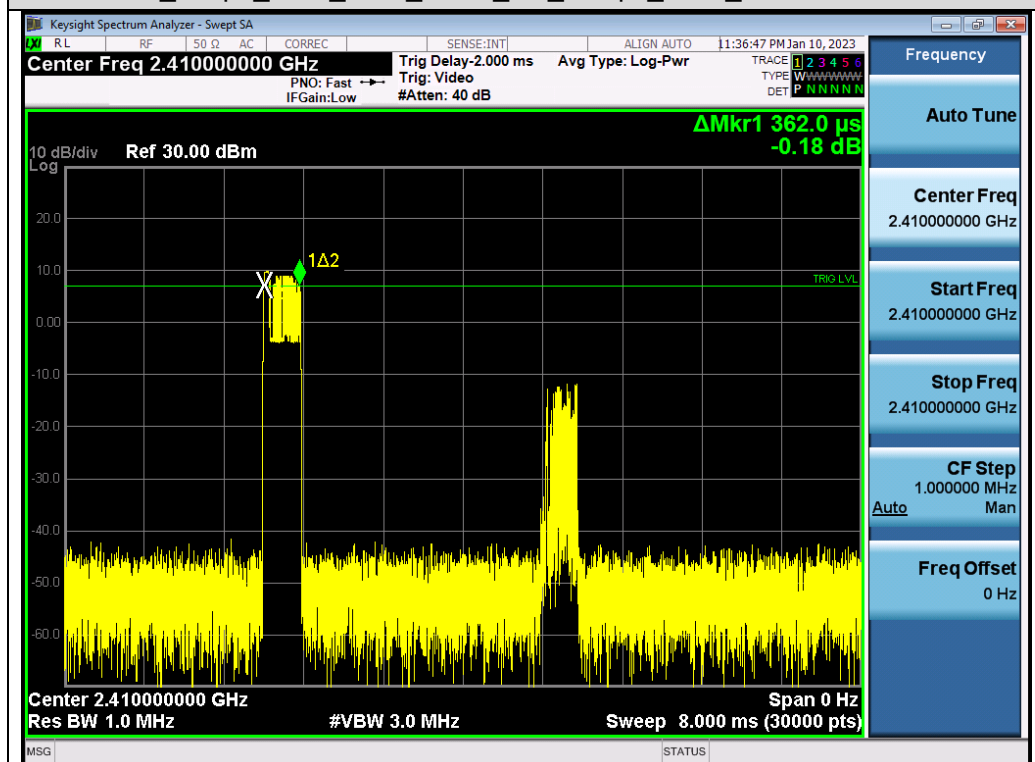
Test_Graph_2.4G_HOP_ANT1_NA_4Mbps_2410_Time per Burst
