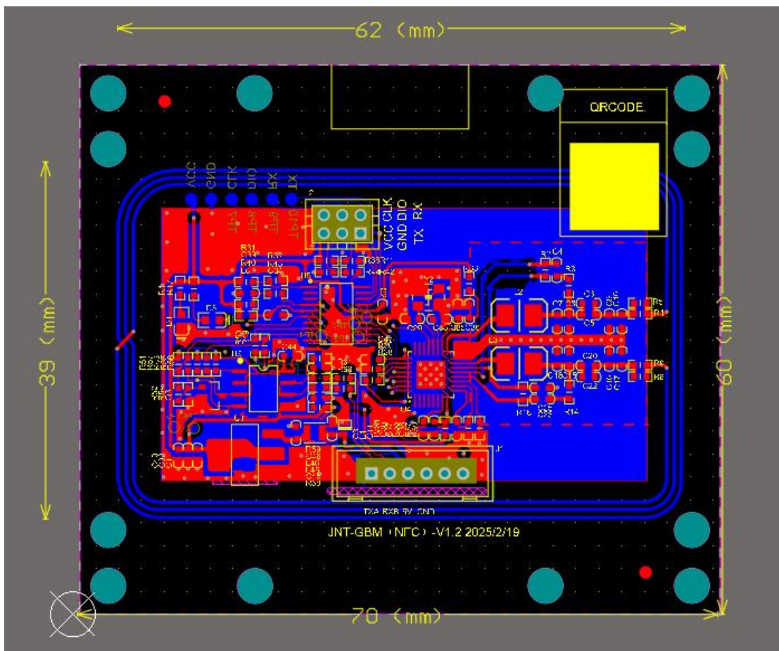
RFID 天线尺寸图
