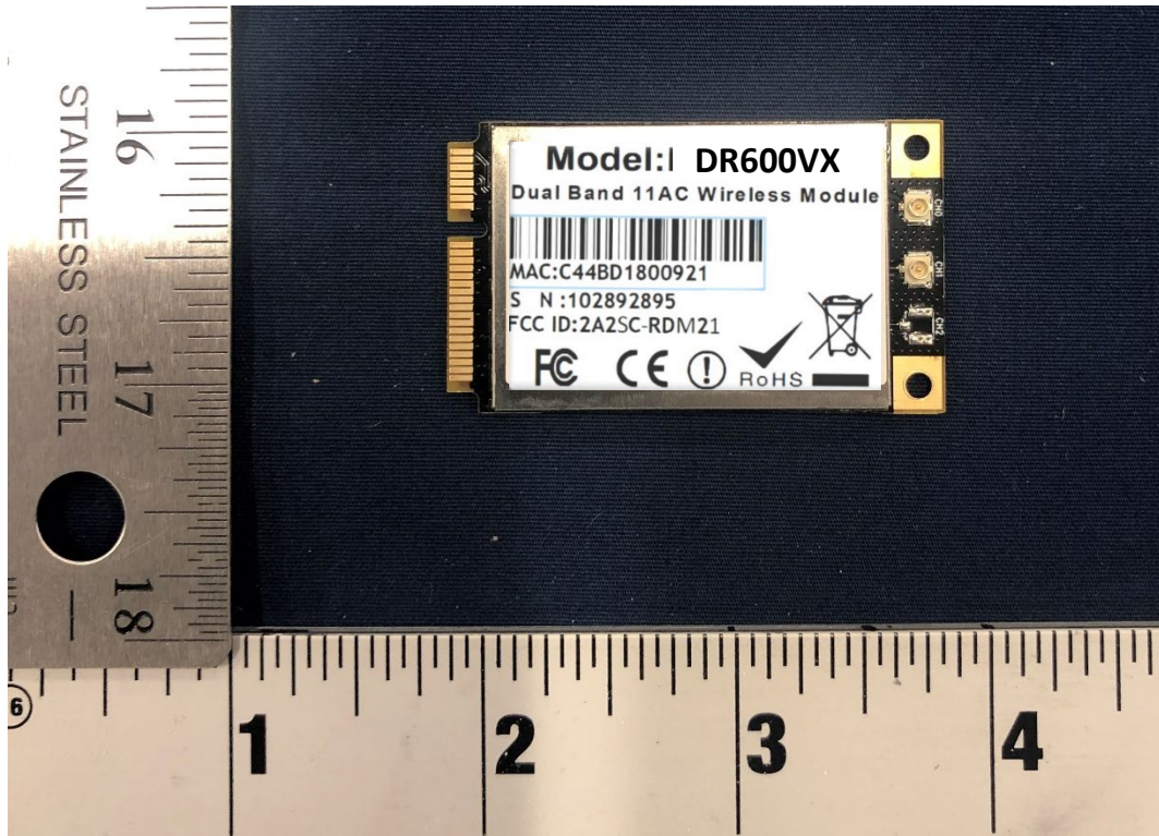
Front of 5 GHz Mini PCIe Radio Module (Radios 1 & 2)
