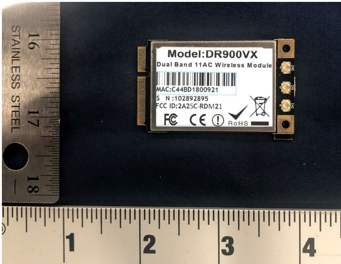
Front of 2.4 GHz Mini PCIe Radio Module (Radio 0)
