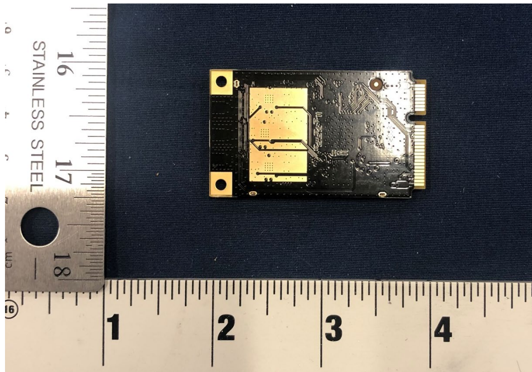
Back of 5 GHz Mini PCIe Radio Module (Radios 1 & 2)
