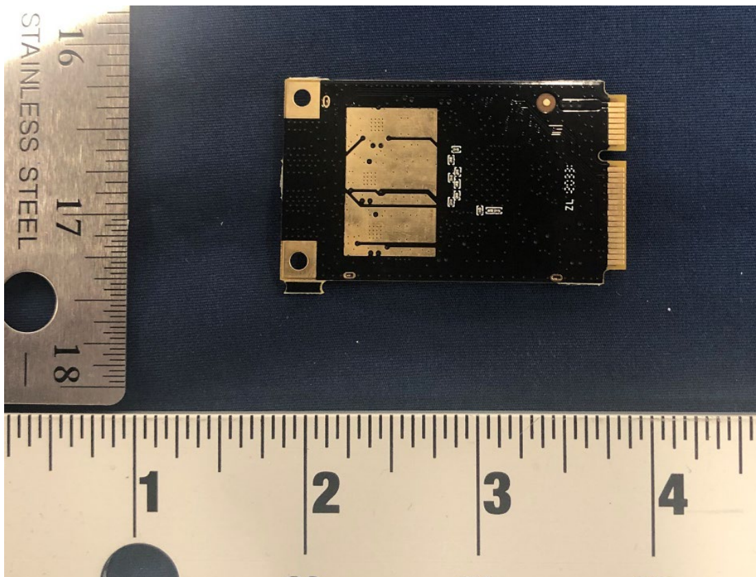
Back of 2.4 GHz Mini PCIe Radio Module (Radio 0)
