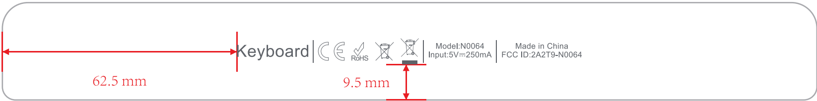
镭雕位置示意，居中
