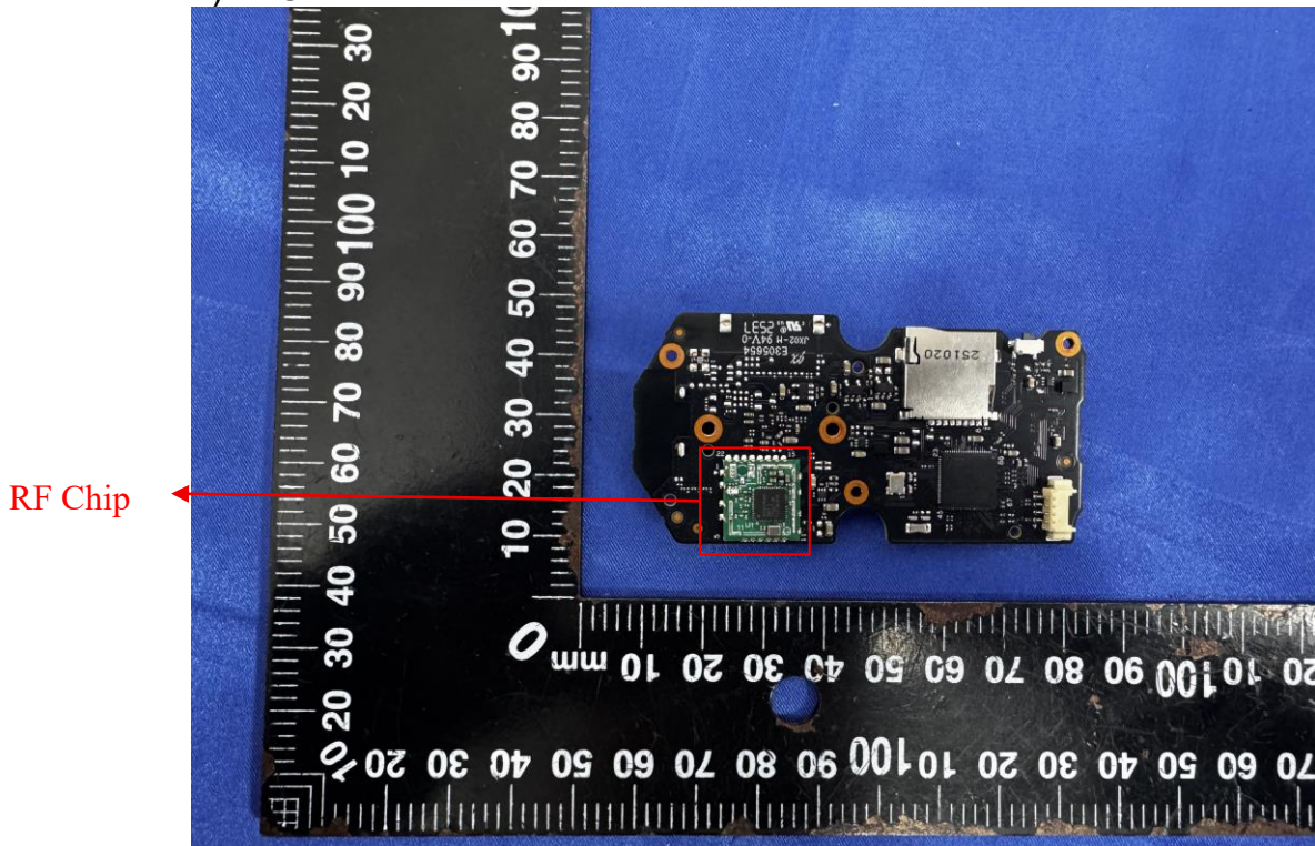
7) EUT Photo
