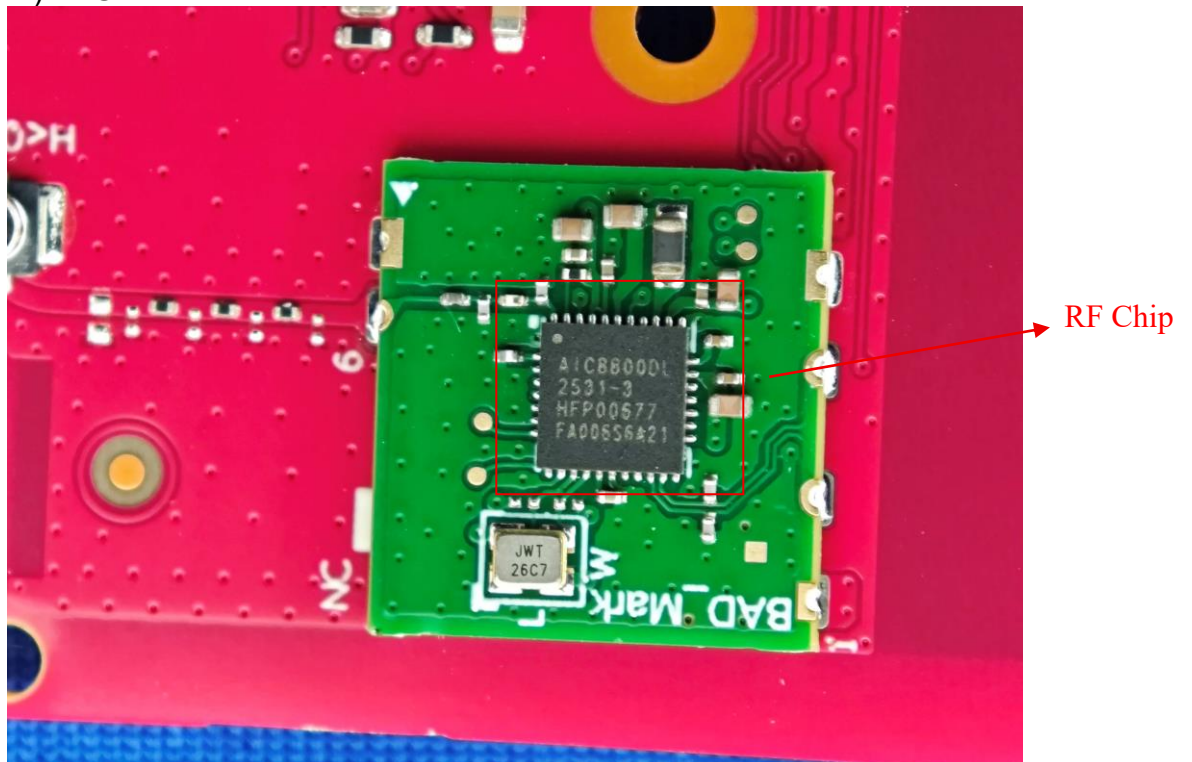
7) EUT Photo
