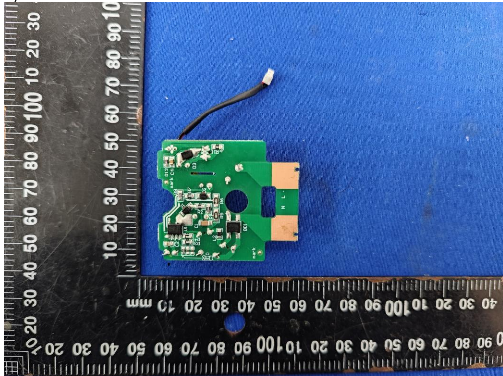
3) EUT Photo
