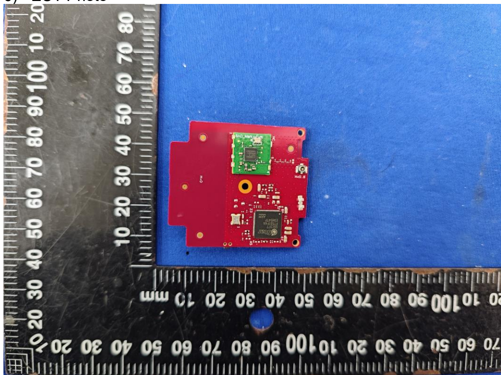
6) EUT Photo
