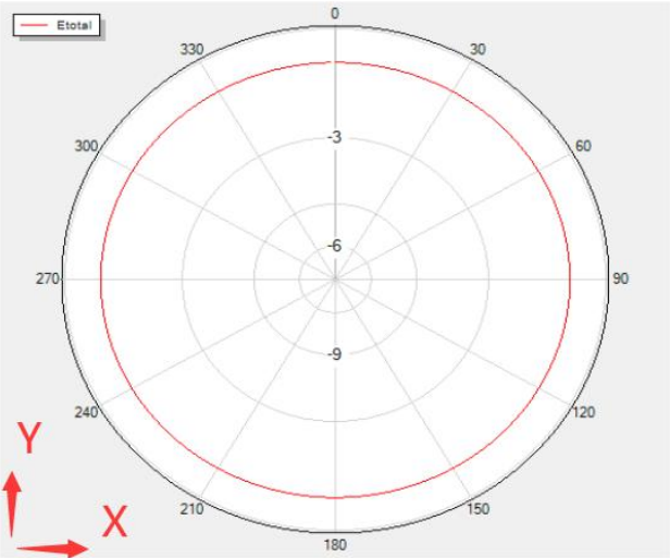
Theta=0 Freq=2460MHz
