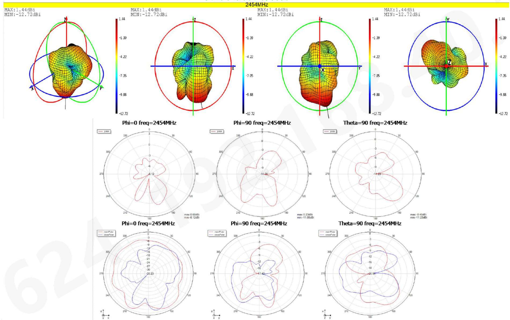
天线苹果图和方向图
