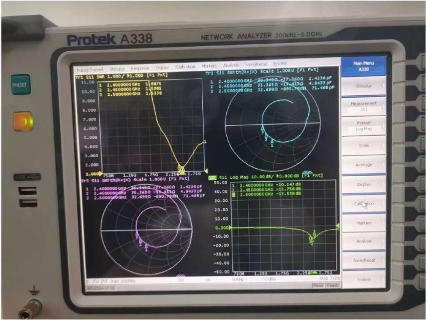
天线smith圆图和S11参数
