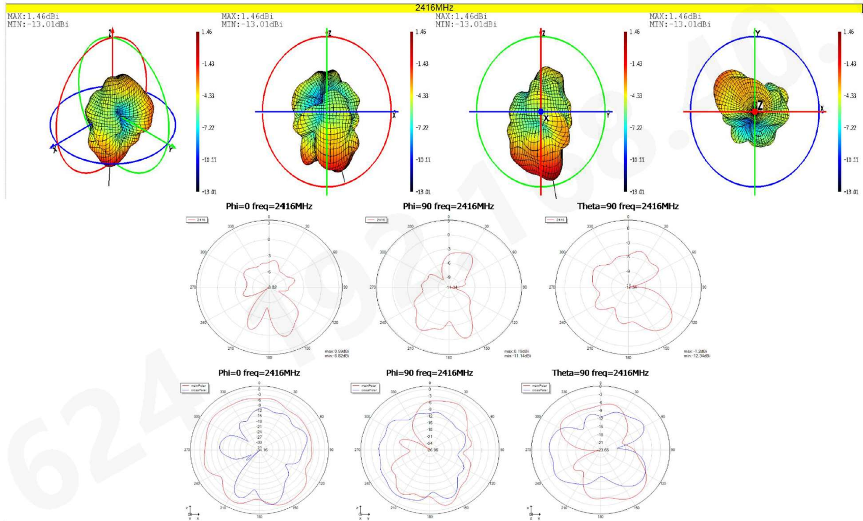
天线苹果图和方向图
