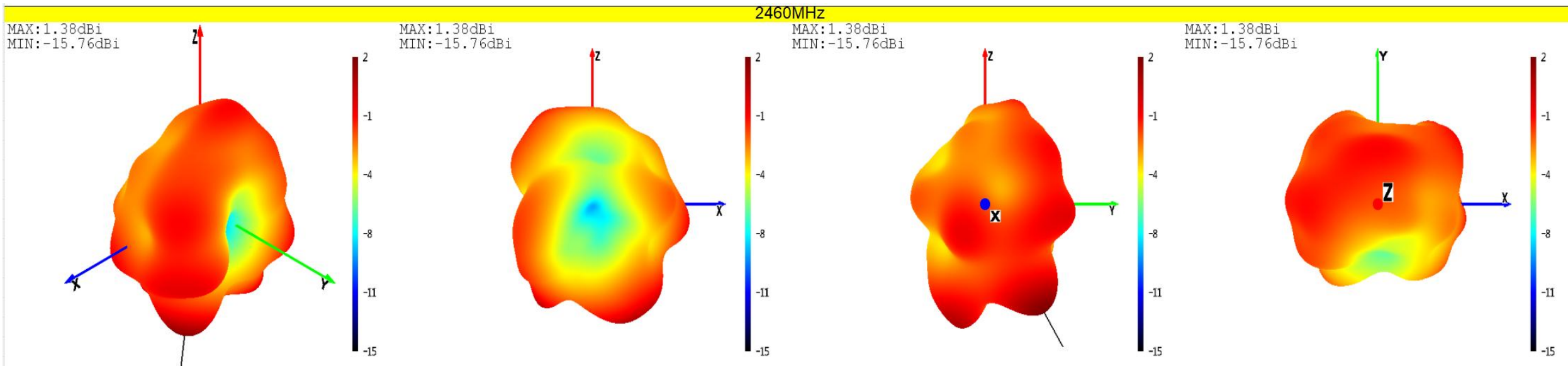
Theta=0 Freq=2460MHz
