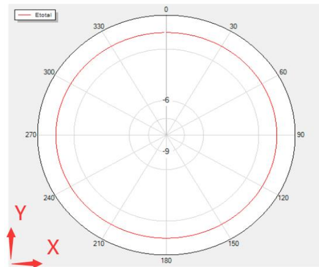
Theta=0 Freq=2428MHz
