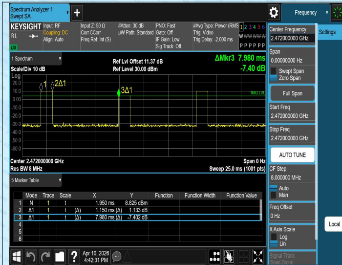
NTVN-TX-Ant1-2472
