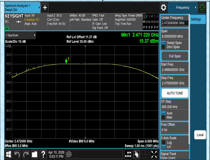
TX-Ant2-2472-PASS
