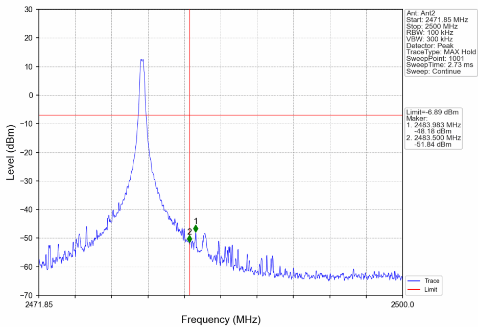
GMSK_HCH_2479.85MHz_Ant2_NTNV
