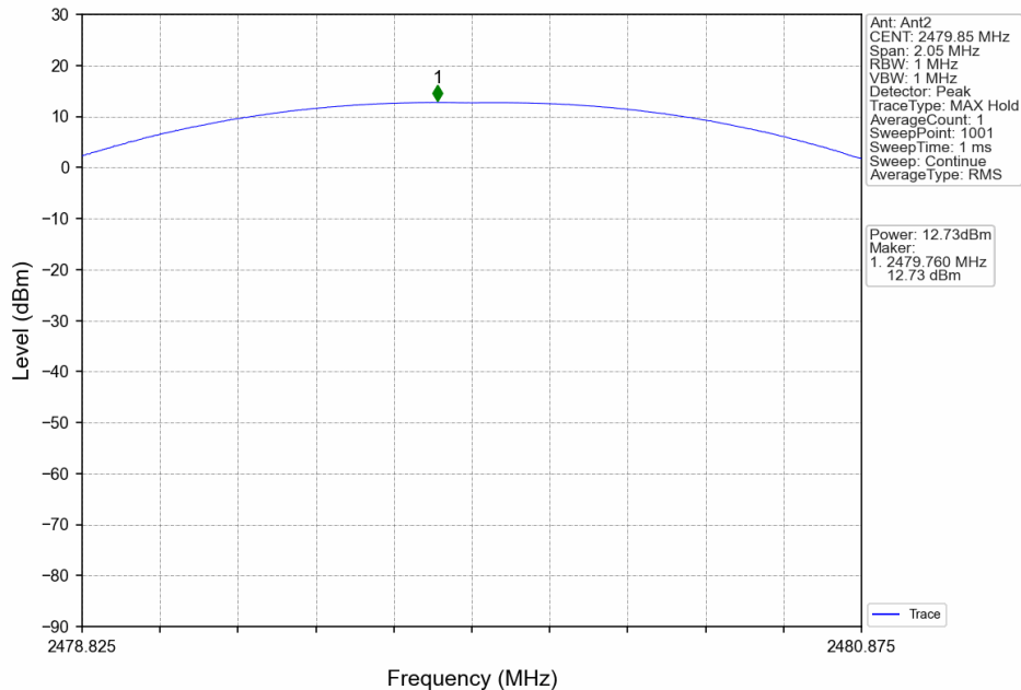
GMSK_HCH_2479.85MHz_Ant2_NTNV
