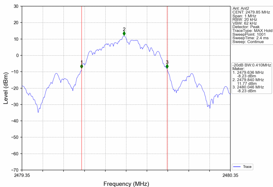
GMSK_HCH_2479.85MHz_Ant2_NTNV
