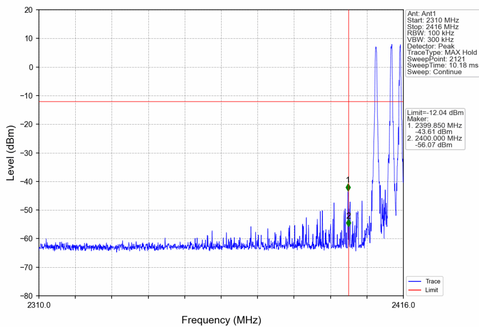
GFSK HOPP_Ant1_NTNV
