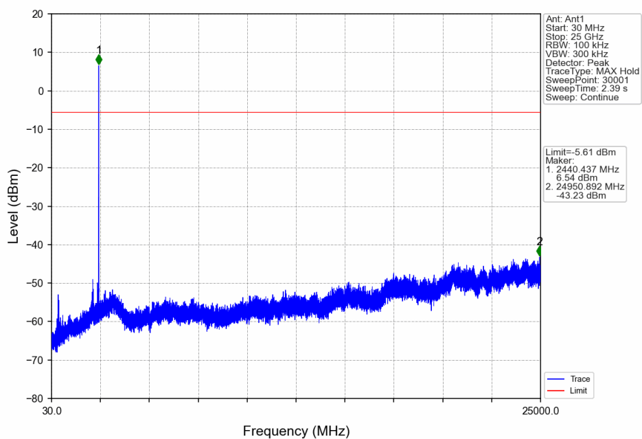
GMSK_MCH_2440MHz_Ant1_NTNV
