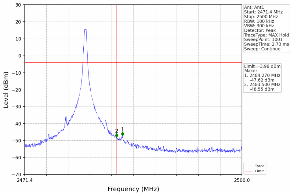
1_HCH_2479.4MHz_Ant1_NTNV
