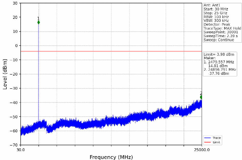
1_HOPP_Ant1_NTNV
