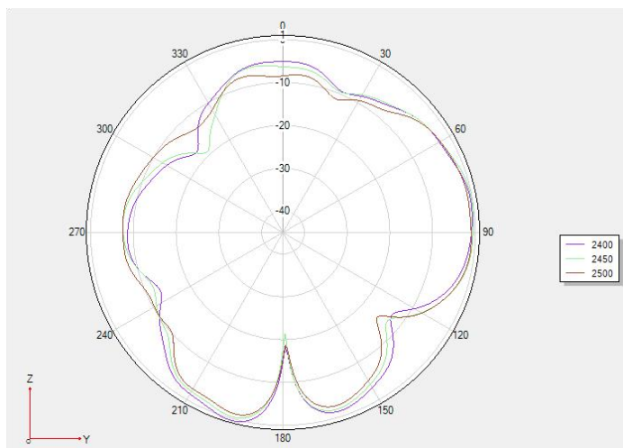
Phi90°2D
