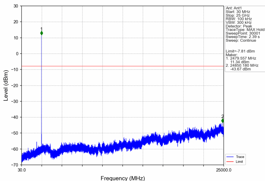
2.4G_HCH_2479.85MHz_Ant1_NTNV
