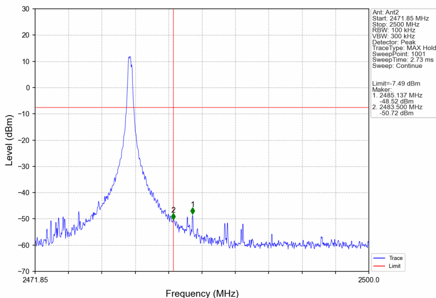
2.4G_HCH_2479.85MHz_Ant2_NTNV
