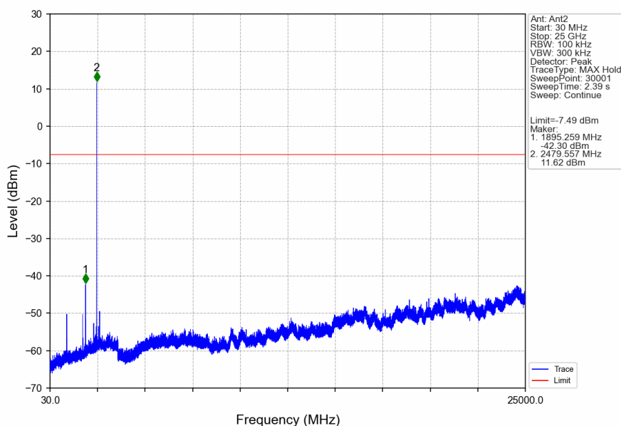
2.4G_HCH_2479.85MHz_Ant2_NTNV
