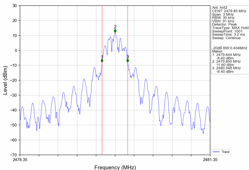
2.4G_HCH_2479.85MHz_Ant2_NTNV
