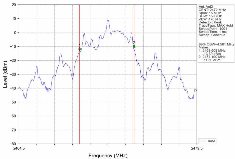
GMSK_HCH_2472MHz_Ant2_NTNV
