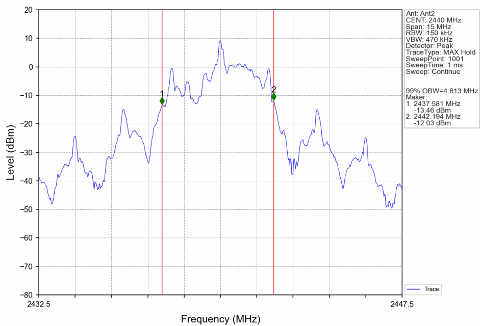
GMSK_MCH_2440MHz_Ant2_NTNV
