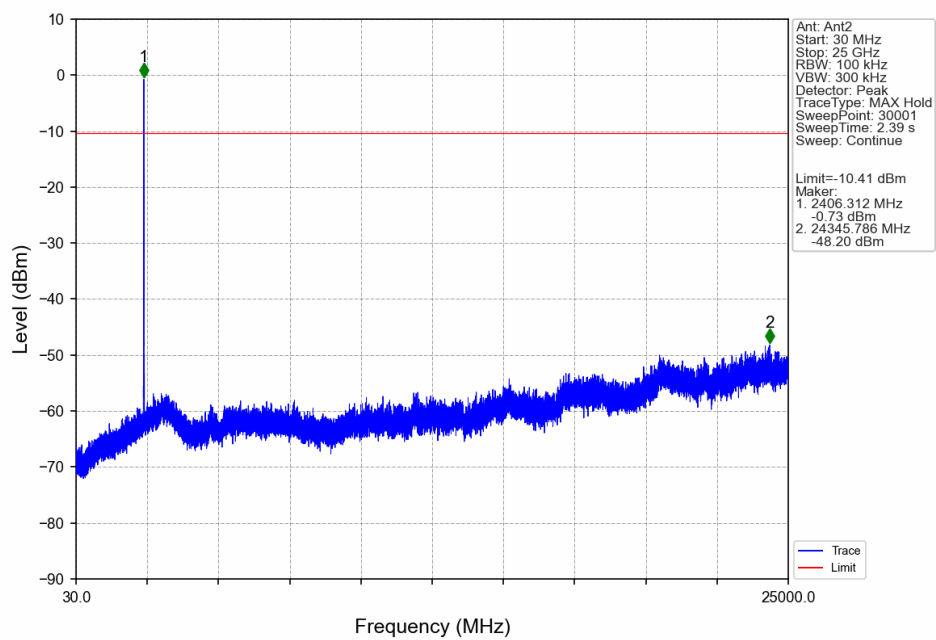
GMSK_LCH_2406MHz_Ant2_NTNV
