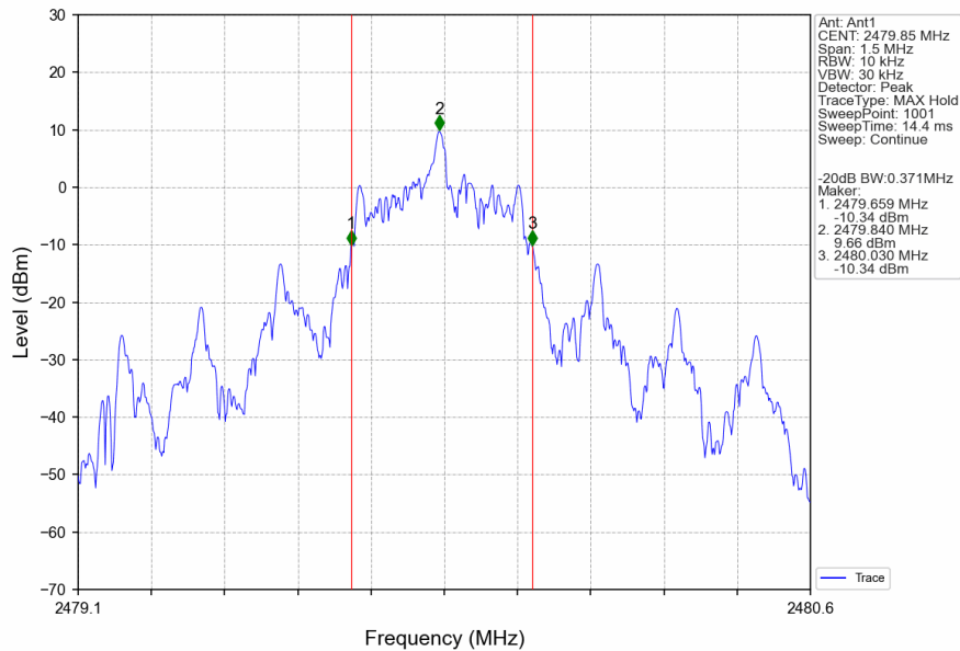
2.4G_HCH_2479.85MHz_Ant1_NTNV
