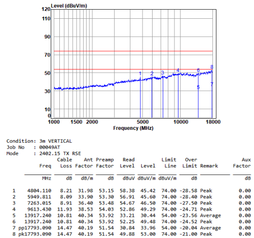
2.4G SRD_TX_CH_L_Vertical
