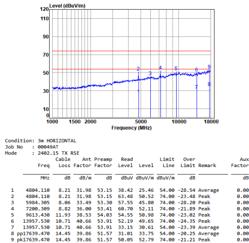
2.4G SRD_TX_CH_L_Horizontal
