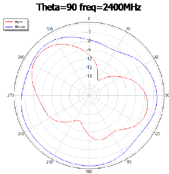
Theta90 ° 面方向图
