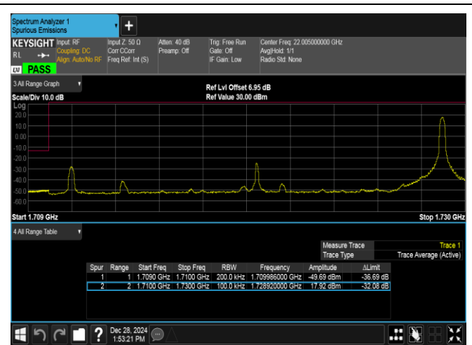
Band4-20MHz-16QAM-20050-1RB#99-PASS
