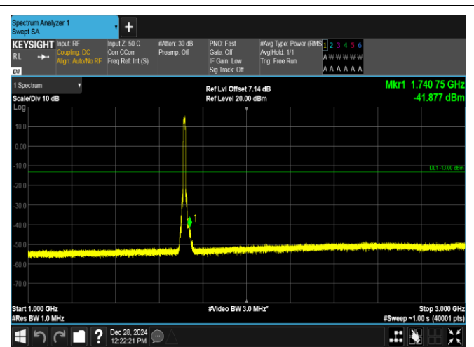
Band4-10MHz-QPSK-20000-50RB#0-1000~3000-PASS
