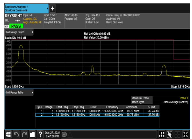
Band25-10MHz-QPSK-26640-1RB#0-PASS
