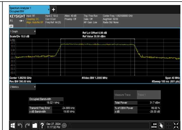
Band25-20MHz-QPSK-26365-100RB#0-PASS
