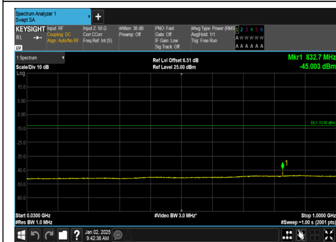
Band4-1513-30~1000MHz-PASS
