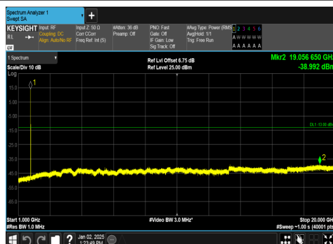
Band4-1413-4-1000~20000MHz-PASS
