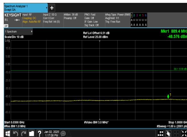
Band4-1312-3-30~1000MHz-PASS
