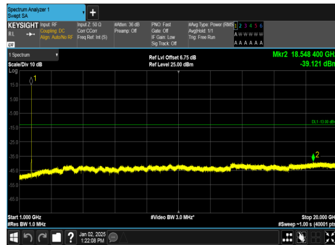
Band4-1312-4-1000~20000MHz-PASS
