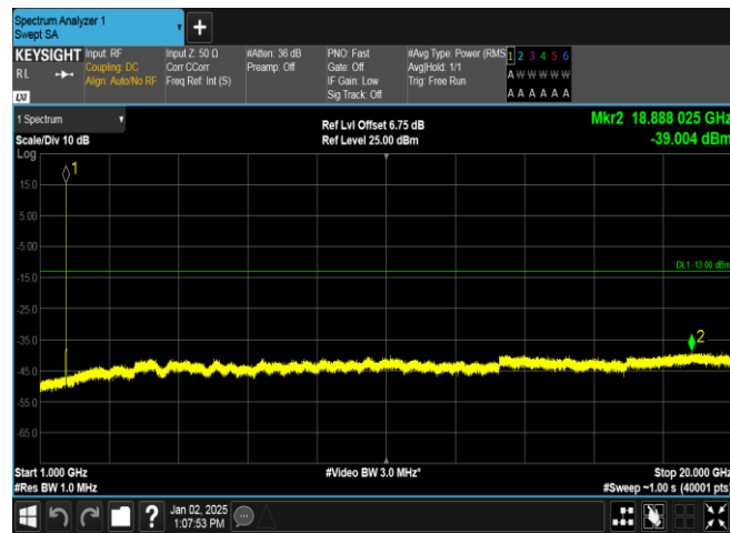
Band4-1312-1-1000~20000MHz-PASS
