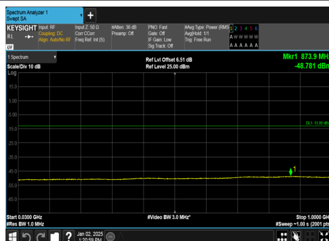
Band4-1513-3-30~1000MHz-PASS
