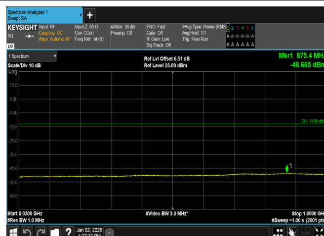
Band4-1413-5-30~1000MHz-PASS
