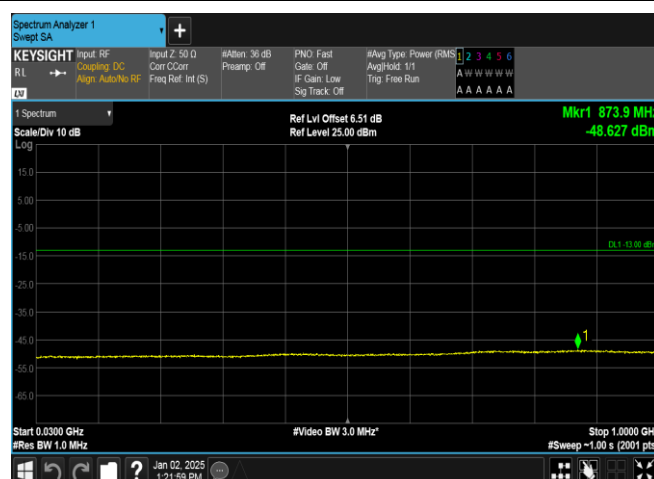
Band4-1312-4-30~1000MHz-PASS
