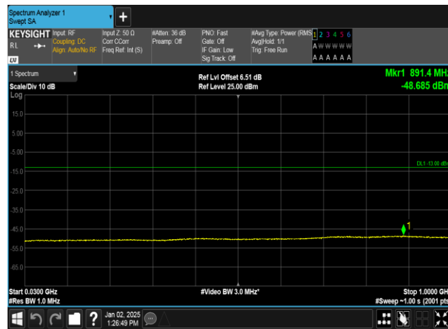
Band4-1312-5-30~1000MHz-PASS
