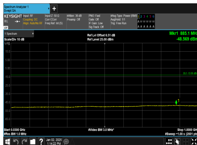
Band4-1413-2-30~1000MHz-PASS
