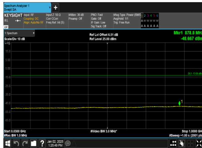
Band4-1513-4-30~1000MHz-PASS
