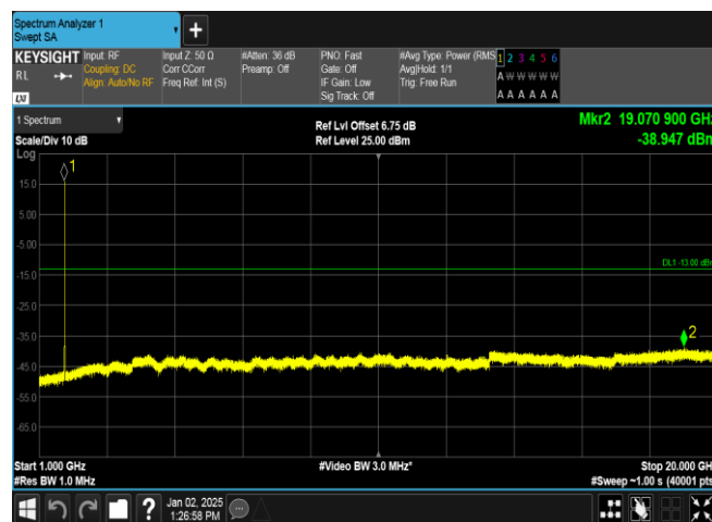
Band4-1312-5-1000~20000MHz-PASS
