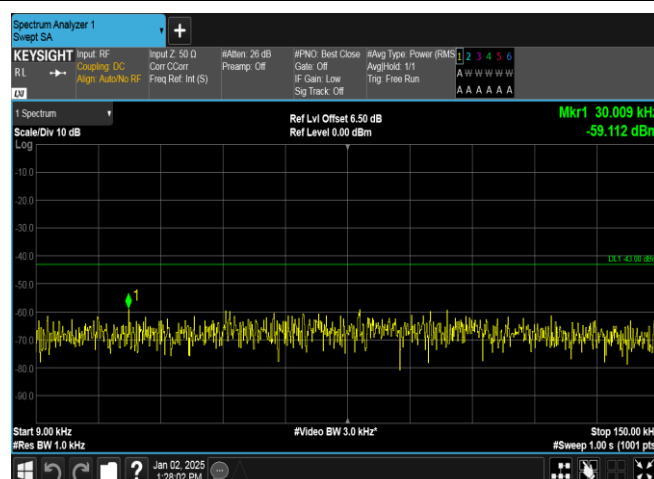
Band4-1513-5-0.009~0.15MHz-PASS
