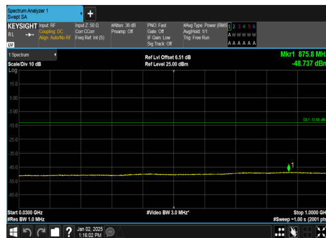
Band4-1513-2-30~1000MHz-PASS
