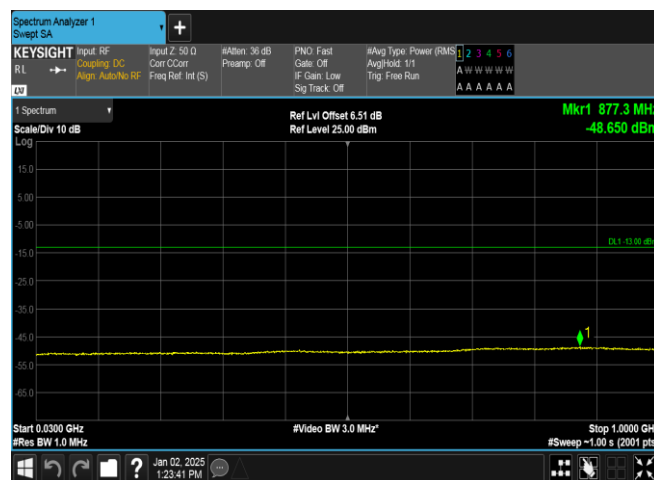
Band4-1413-4-30~1000MHz-PASS
