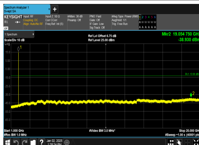
Band4-1513-5-1000~20000MHz-PASS
