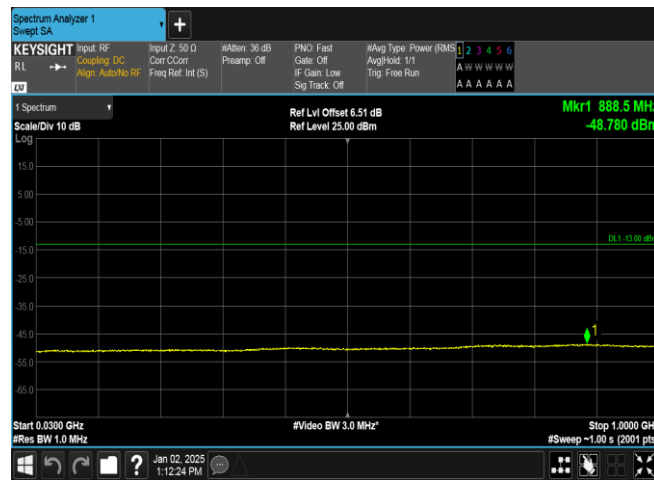
Band4-1312-2-30~1000MHz-PASS
