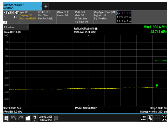
Band4-1413-3-30~1000MHz-PASS
