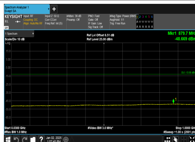
Band4-1312-1-30~1000MHz-PASS
