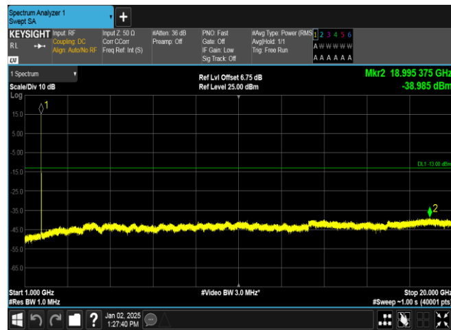
Band4-1413-5-1000~20000MHz-PASS
