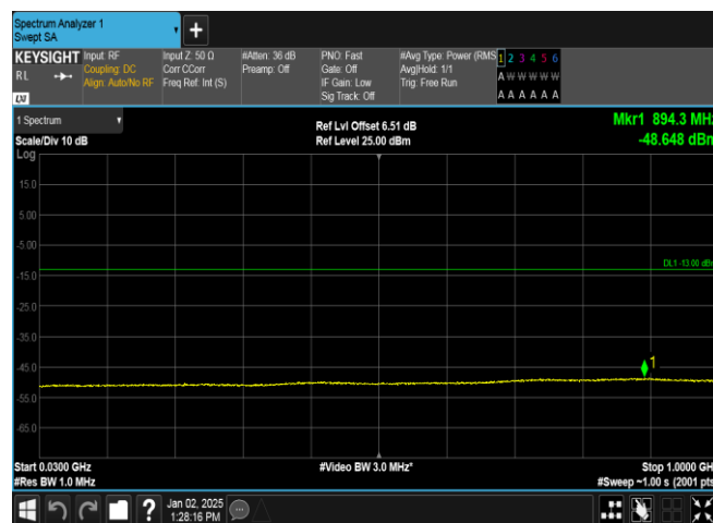
Band4-1513-5-30~1000MHz-PASS
