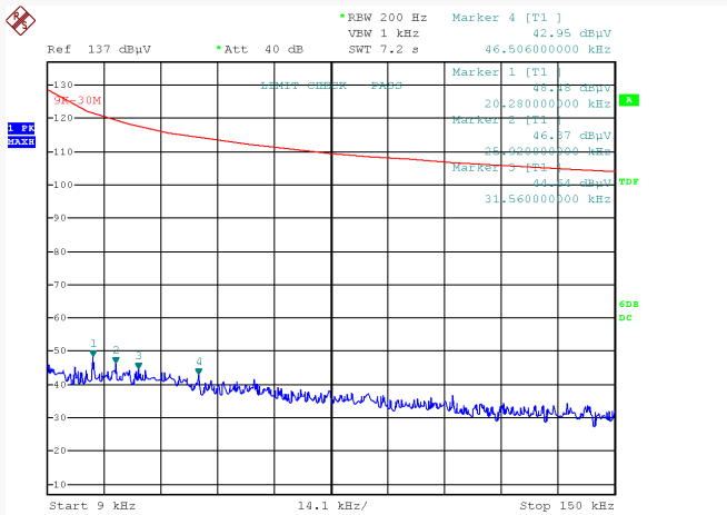
9kHz-150kHz
