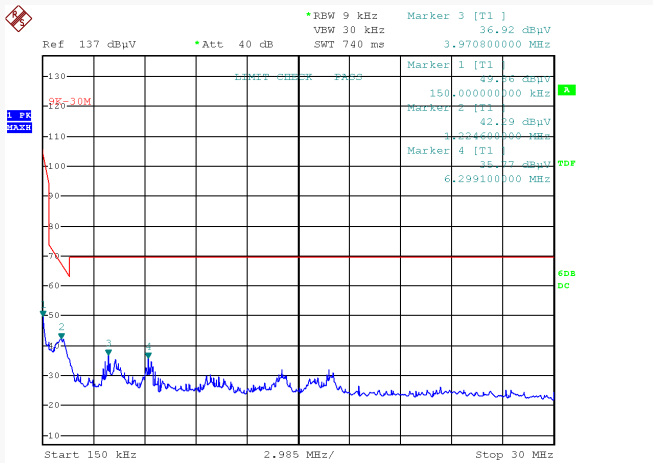
150kHz-30MHz
