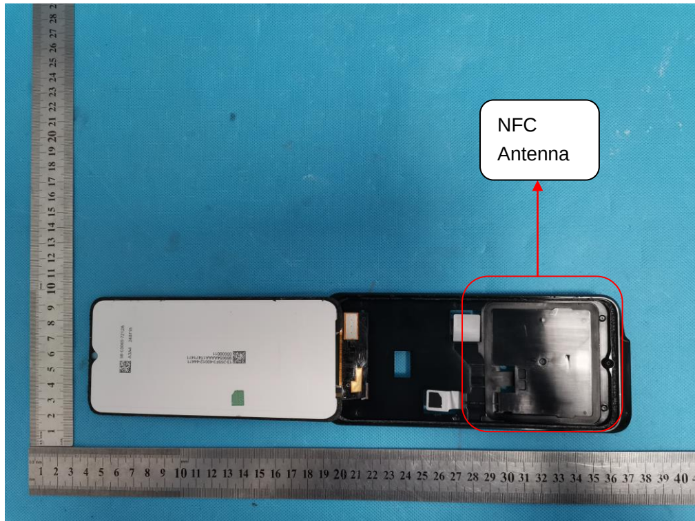
NFC ANTENNA
