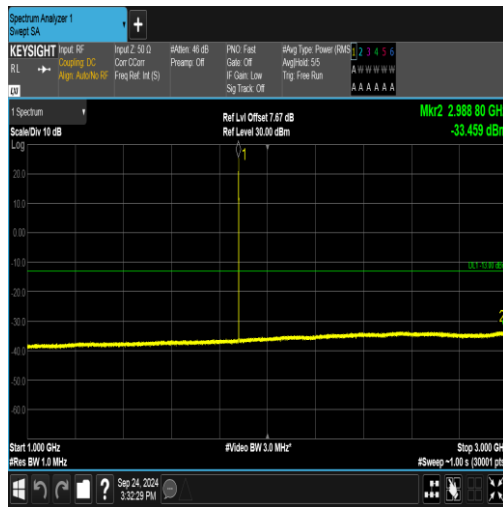
GSM1900-661-0-1000~3000MHz-PASS
