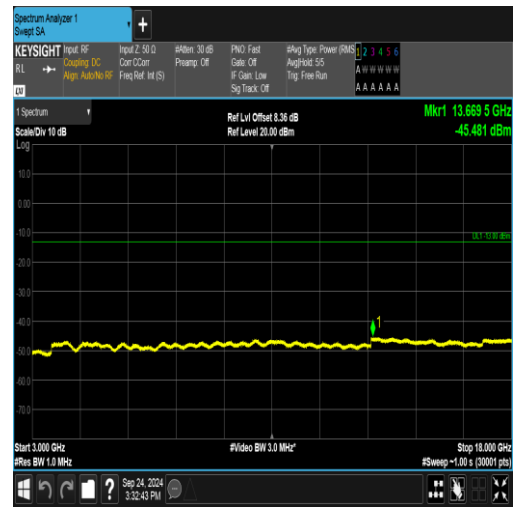
GSM1900-661-0-3000~18000MHz-PASS
