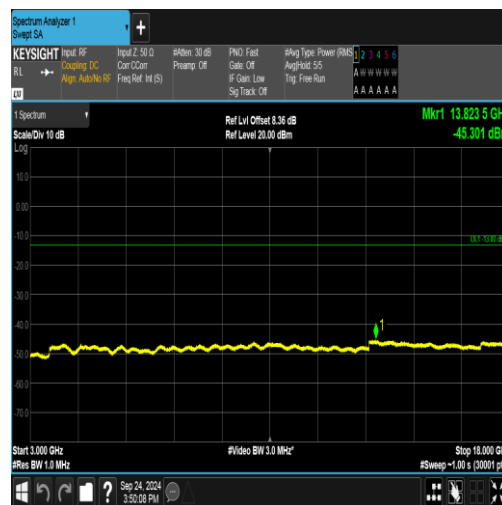
GPRS1900-810-0-3000~18000MHz-PASS
