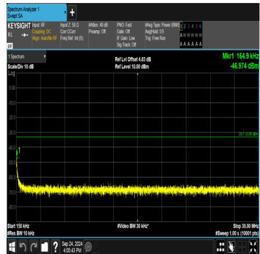
EGPRS1900-810-2-0.15~30MHz-PASS
