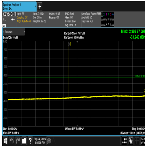
EGPRS1900-661-2-1000~3000MHz-PASS
