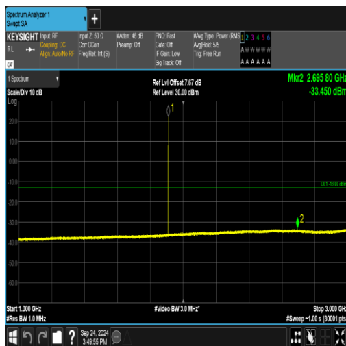
GPRS1900-810-0-1000~3000MHz-PASS
