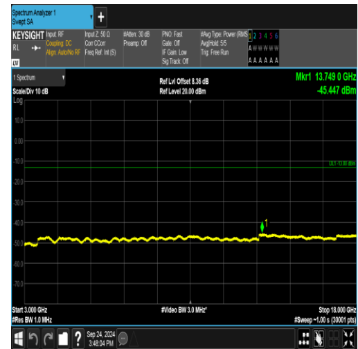
GPRS1900-512-0-3000~18000MHz-PASS
