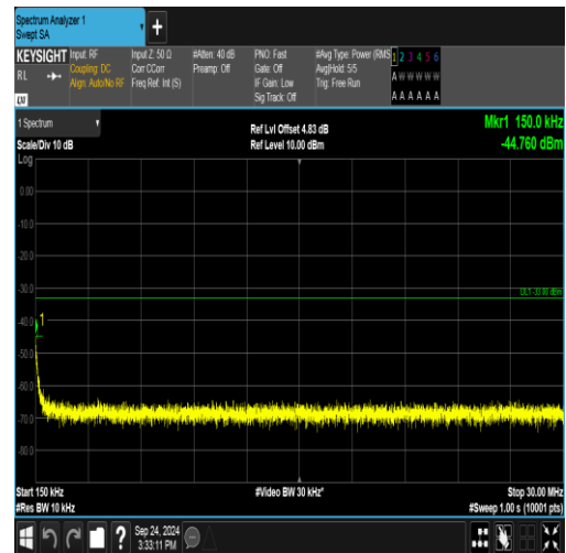
GSM1900-810-0-0.15~30MHz-PASS
