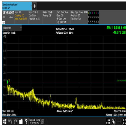
GSM1900-810-0-0.009~0.15MHz-PASS
