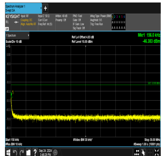
GPRS1900-661-0-0.15~30MHz-PASS
