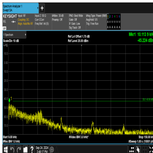
GPRS1900-661-0-0.009~0.15MHz-PASS
