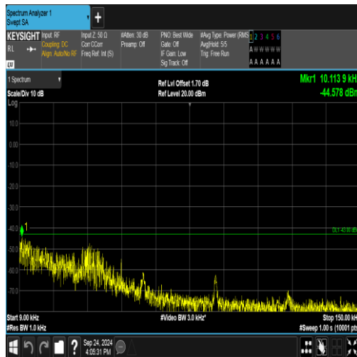
EGPRS1900-810-2-0.009~0.15MHz-PASS
