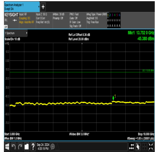
EGPRS1900-661-2-3000~18000MHz-PASS
