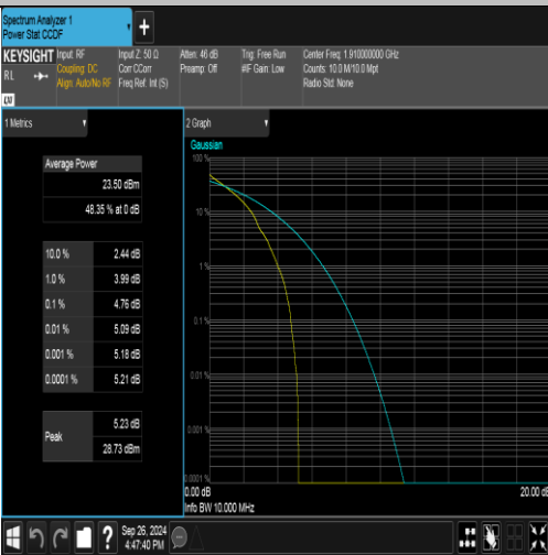
Band25-10MHz-QPSK-26640-1RB#0-PASS
