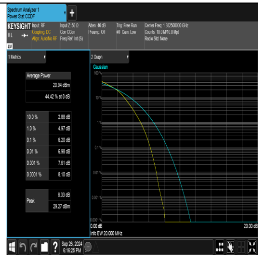
Band25-20MHz-16QAM-26365-100RB#0-PASS
