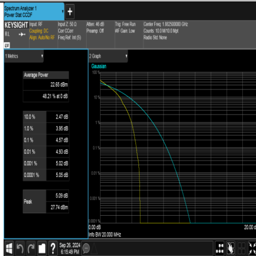
Band25-20MHz-QPSK-26365-1RB#0-PASS
