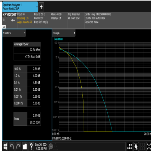
Band25-5MHz-QPSK-26365-1RB#0-PASS
