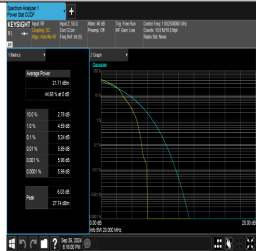
Band25-20MHz-16QAM-26365-1RB#0-PASS
