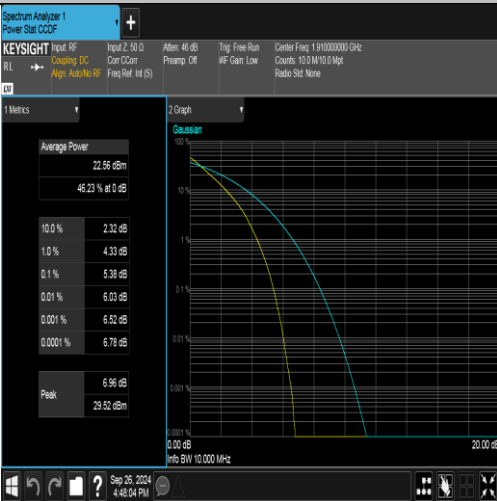
Band25-10MHz-QPSK-26640-50RB#0-PASS
