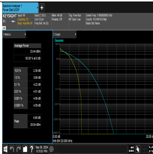
Band25-20MHz-QPSK-26140-1RB#0-PASS
