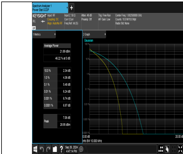
Band25-10MHz-QPSK-26365-50RB#0-PASS
