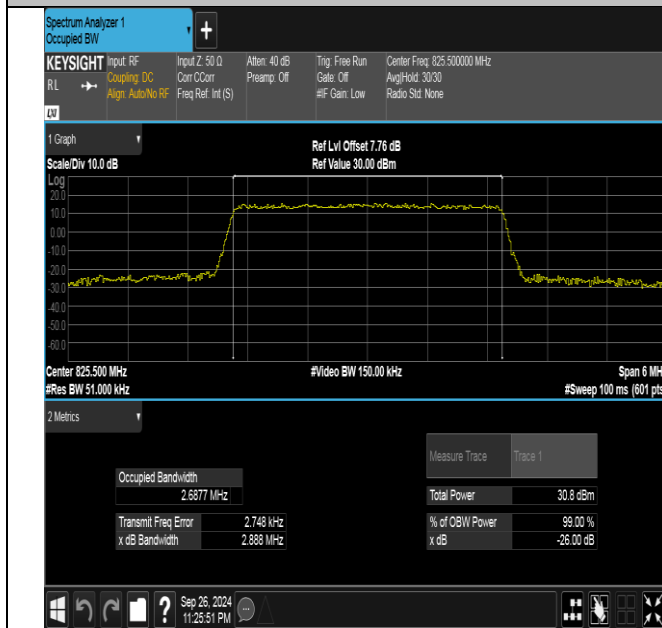
Band26(824-849)-3MHz-QPSK-26805-15RB#0-PASS
