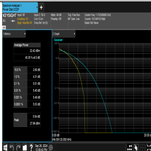
Band4-20MHz-QPSK-20175-1RB#0-PASS
