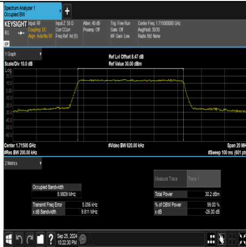
Band4-10MHz-QPSK-20000-50RB#0-PASS
