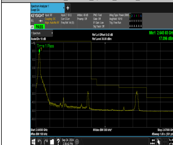
Band41_10MHz_QPSK_41190_1RB#0
