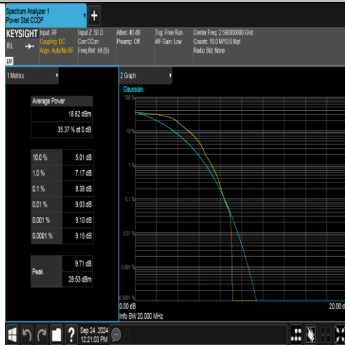
Band41(2535-2655)-20MHz-QPSK-40590-1RB#0-PASS
