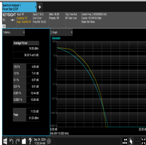
Band41(2535-2655)-10MHz-QPSK-41190-50RB#0-PASS
