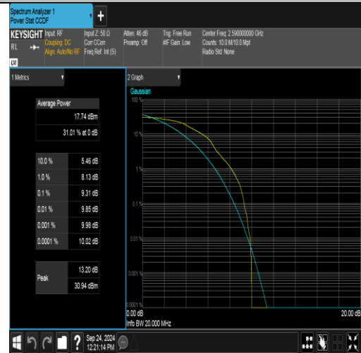
Band41(2535-2655)-20MHz-16QAM-40590-1RB#0-PASS
