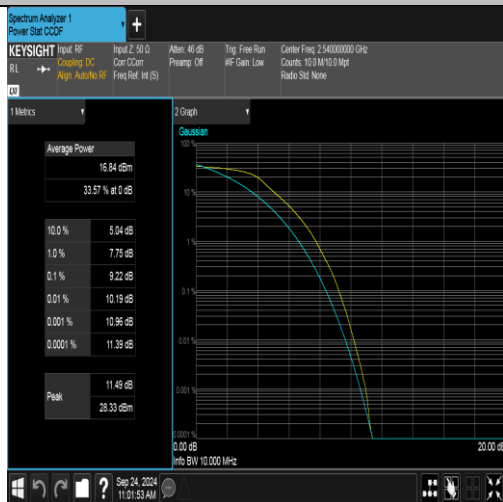
Band41(2535-2655)-10MHz-QPSK-40090-50RB#0-PASS
