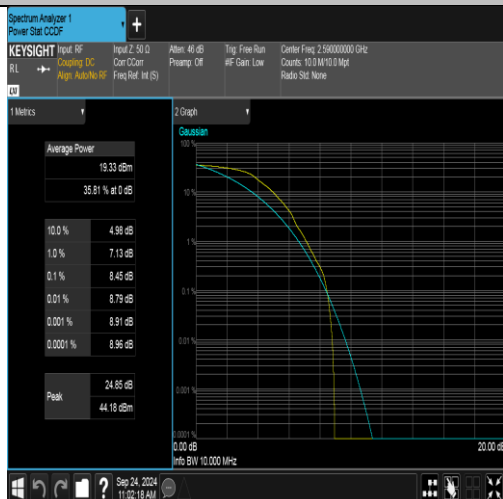
Band41(2535-2655)-10MHz-QPSK-40590-1RB#0-PASS
