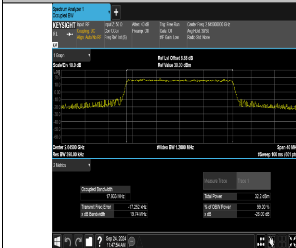
Band41(2535-2655)-20MHz-QPSK-41140-100RB#0-PASS
