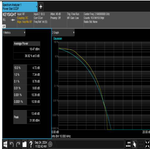
Band41(2535-2655)-10MHz-QPSK-40590-50RB#0-PASS
