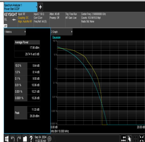
Band41(2535-2655)-10MHz-16QAM-40590-1RB#0-PASS
