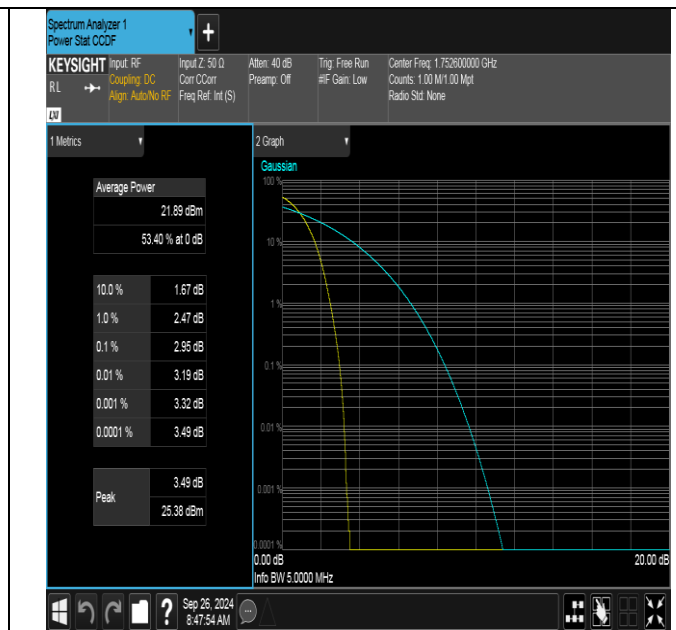
Band4-1513-PASS
