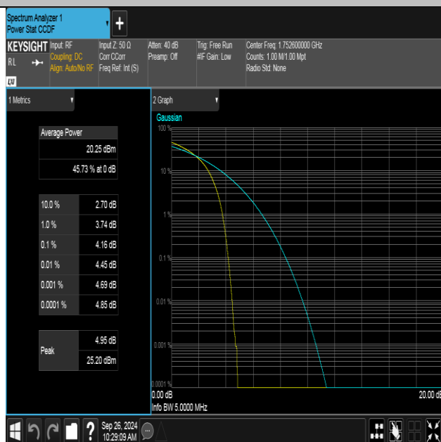
Band4-1513-5-PASS
