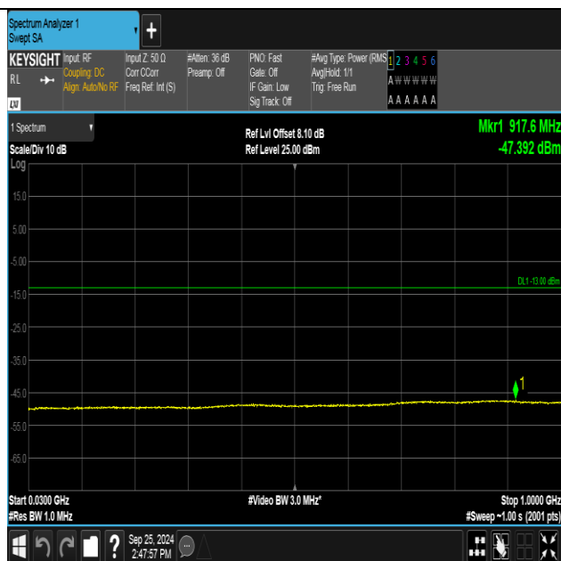
Band2-9400-3-30~1000MHz-PASS
