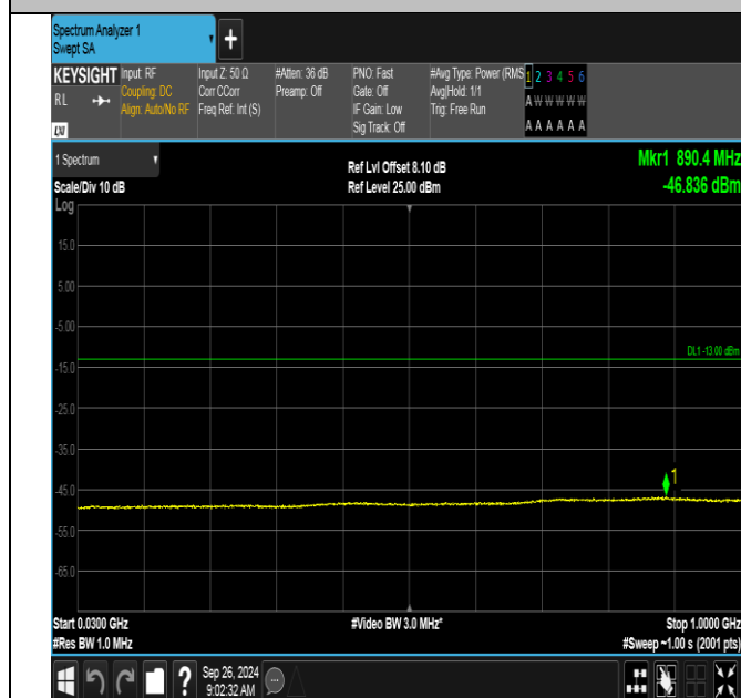
Band4-1413-30~1000MHz-PASS
