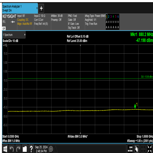
Band2-9538-3-30~1000MHz-PASS
