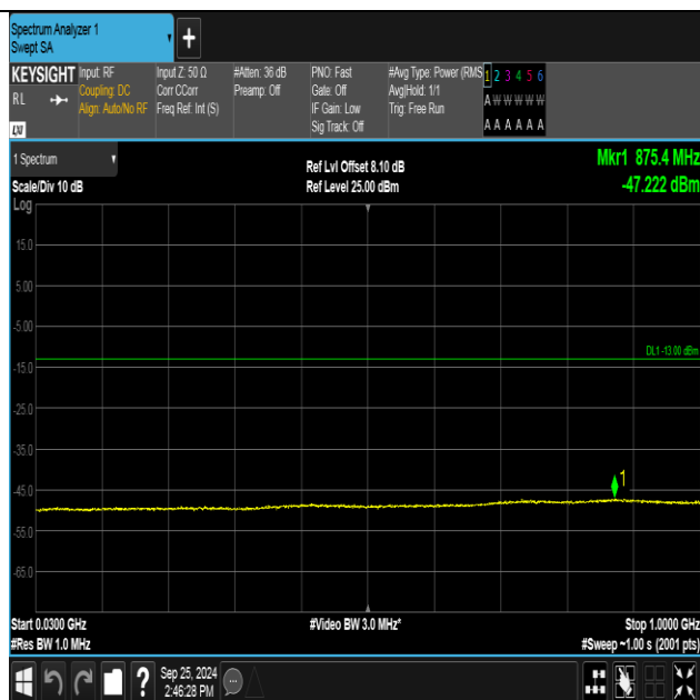
Band2-9538-2-30~1000MHz-PASS
