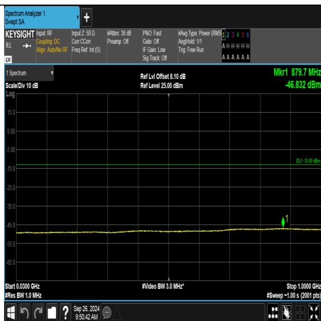
Band4-1513-3-30~1000MHz-PASS
