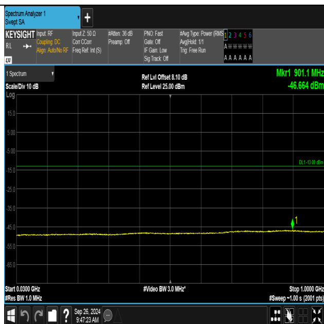
Band4-1312-2-30~1000MHz-PASS
