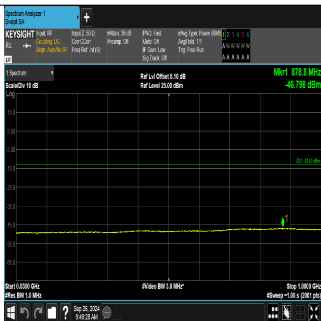
Band4-1312-3-30~1000MHz-PASS
