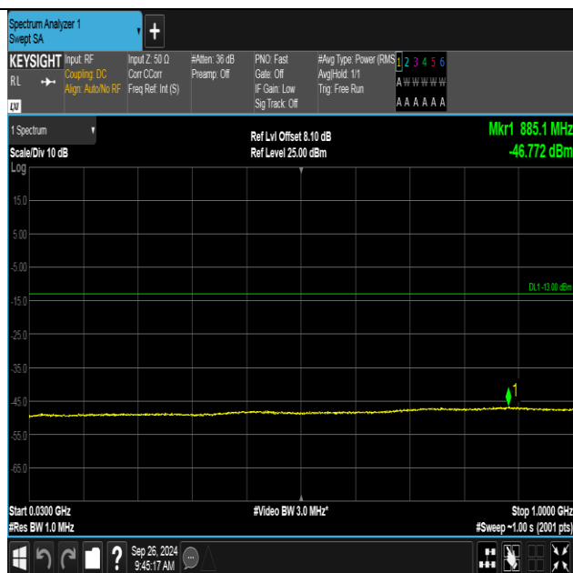
Band4-1312-1-30~1000MHz-PASS
