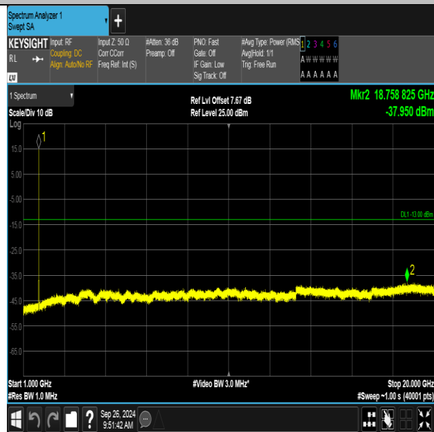
Band4-1312-4-1000~20000MHz-PASS
