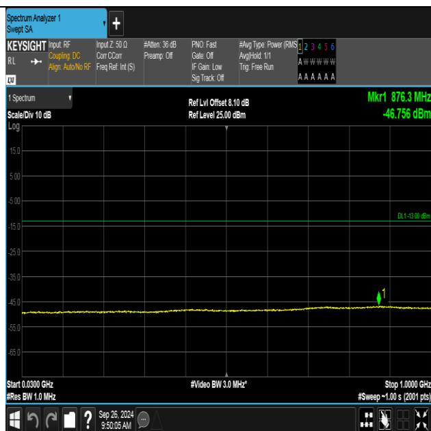
Band4-1413-3-30~1000MHz-PASS
