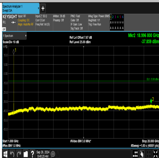
Band4-1312-1-1000~20000MHz-PASS
