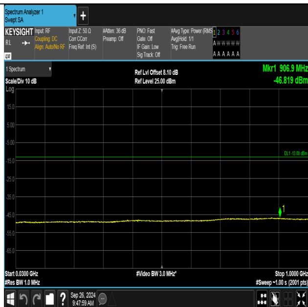
Band4-1413-2-30~1000MHz-PASS
