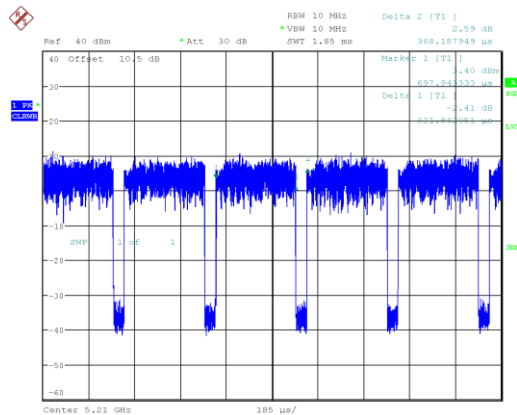
802.11ac80 mode
