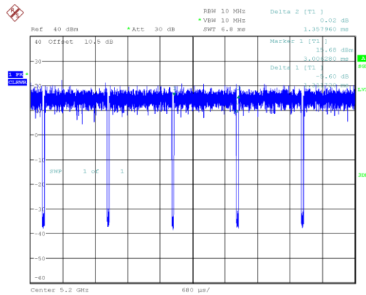
802.11ac20 mode
