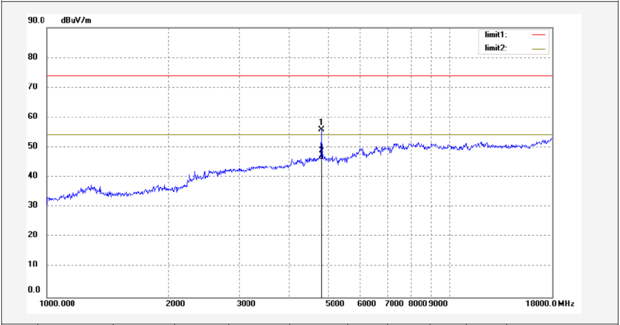
BLE Low Channel Horizontal
