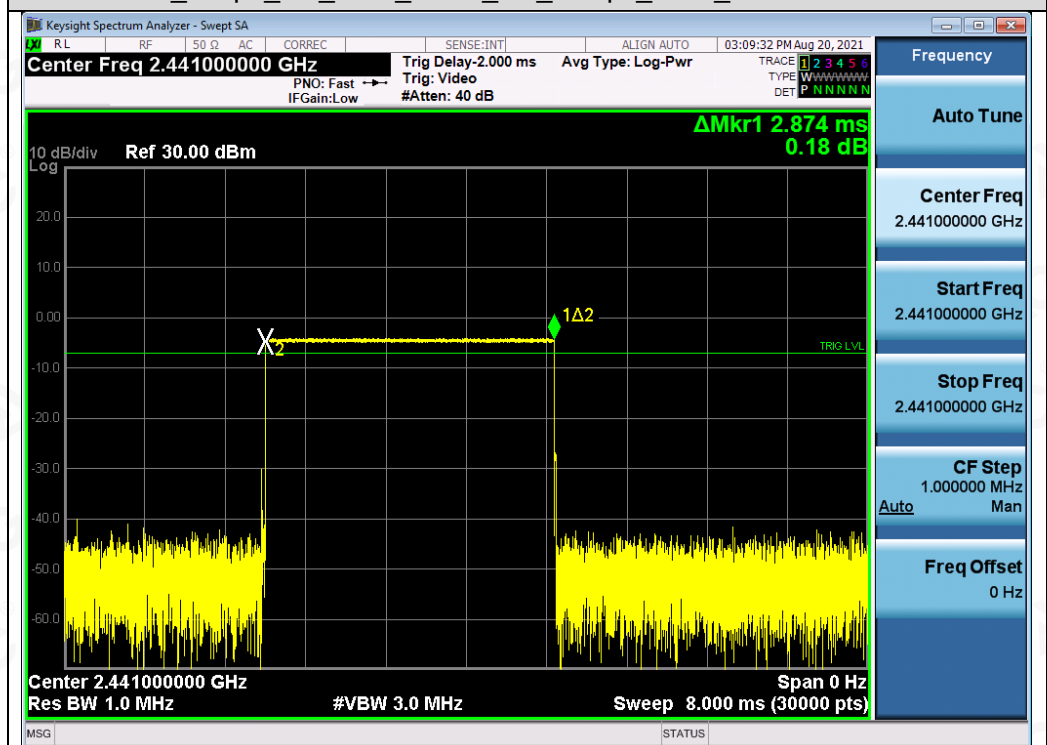
Test_Graph_BR_HOP_ANT1_NA_1Mbps_2441_Time per Burst
