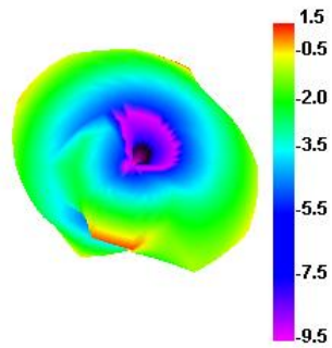
2400.000MHz E1
