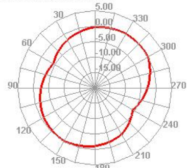
2450.000MHz H
