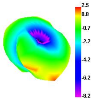
2450.000MHz E1
