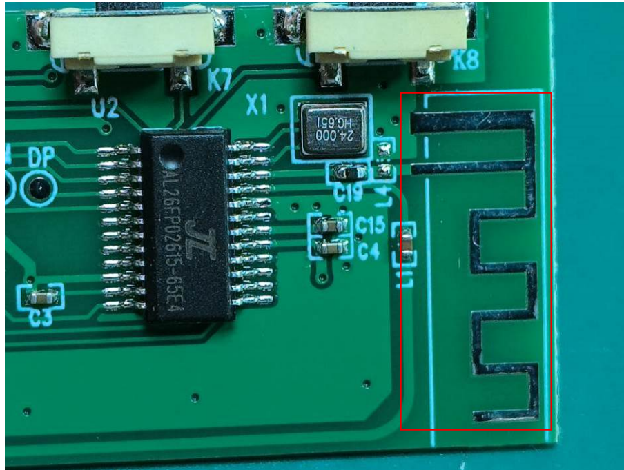
BT ANT
