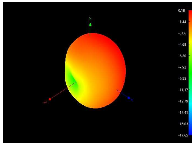
2500MHz 3D
