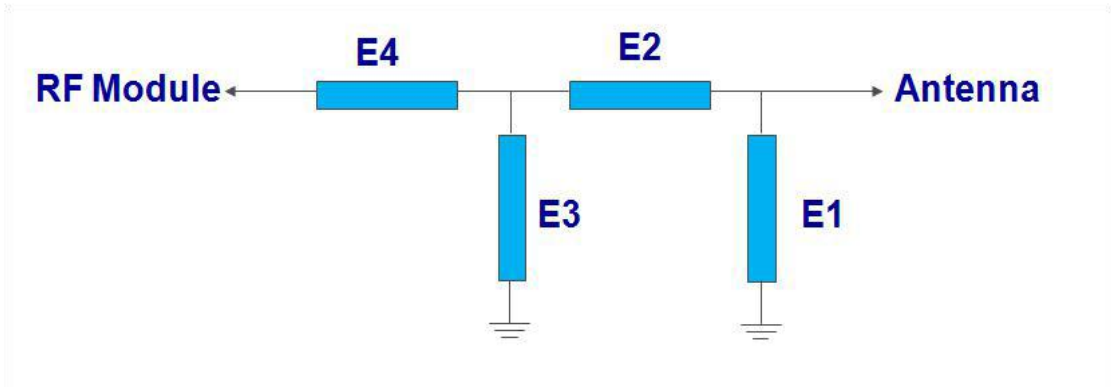
匹配电路
