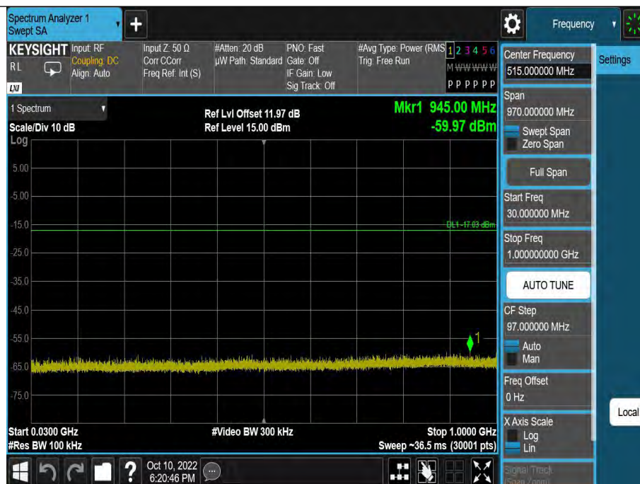
DH5-Ant1-2441-30~1000-2.97
